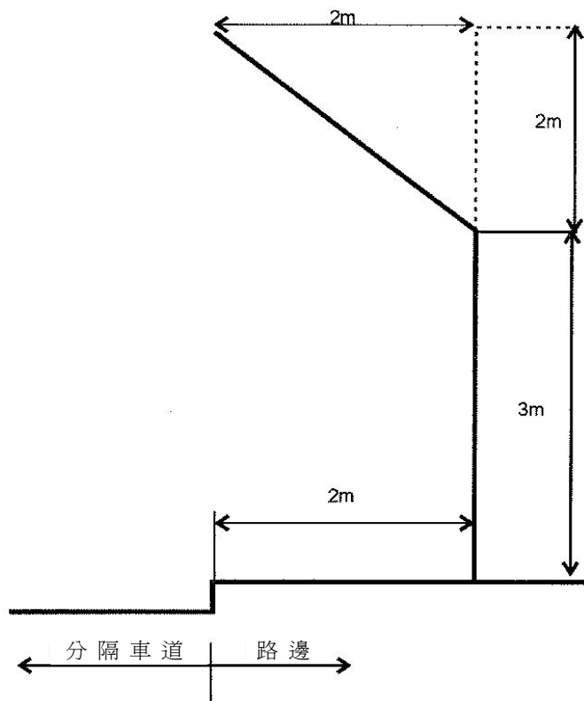
建議在屯門第54區 D7 路設置的懸臂式隔音屏障
