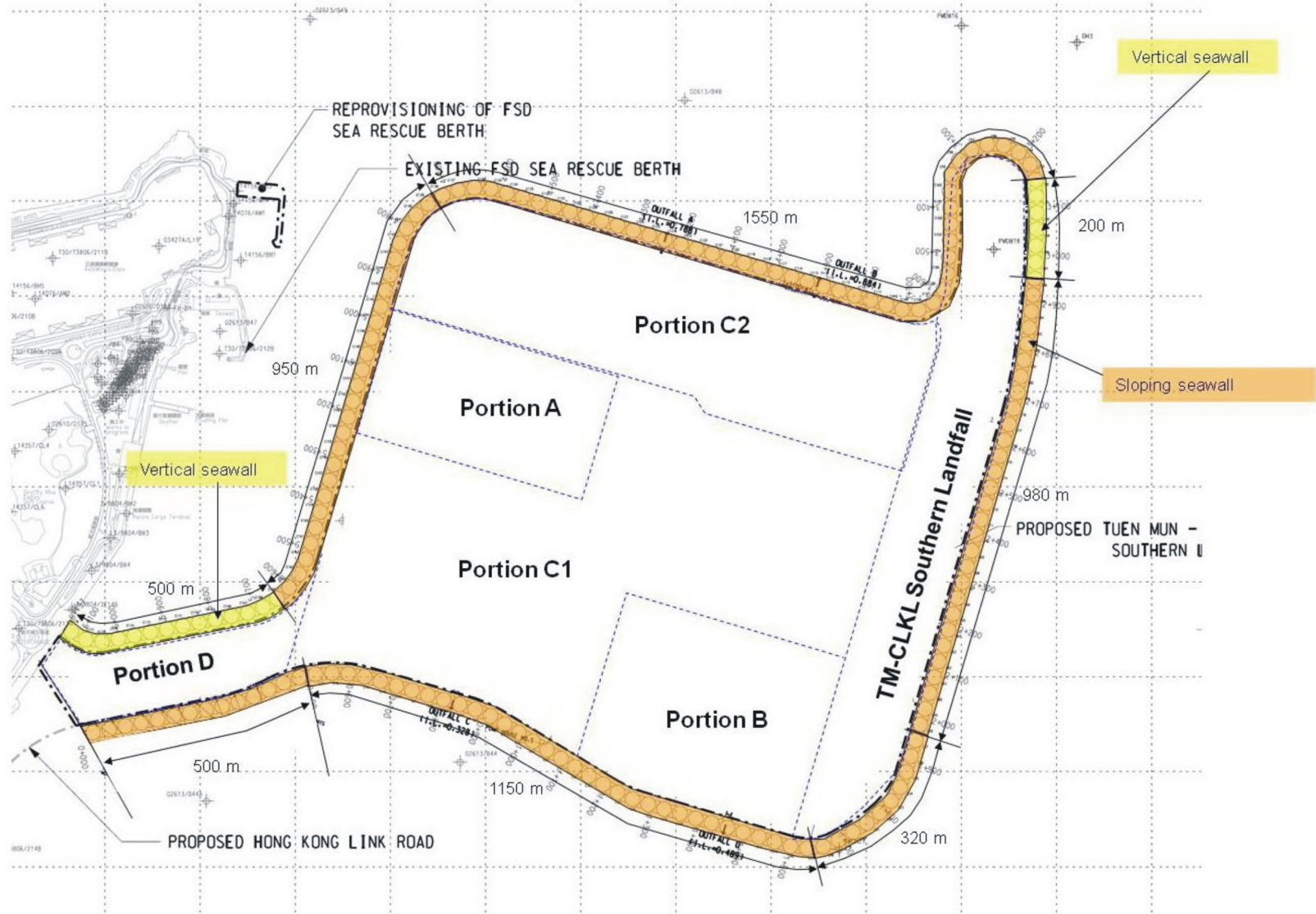
Figure 28 - Location Plan for Vertical Seawalls and Sloping Seawalls 圖 28 - 垂直海堤及坡海堤位置圖 (Plan originated from Figure 2.8 of submitted documents dated 11 June 2010 with Application for Variation of an Environmental Permit no. VEP-315/2010) (圖則源自於2010年6月11日提交更改環境許可證申請編號VEP-315/2010的文件 圖2.8)
