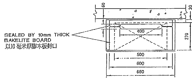
橫切面 B-B
