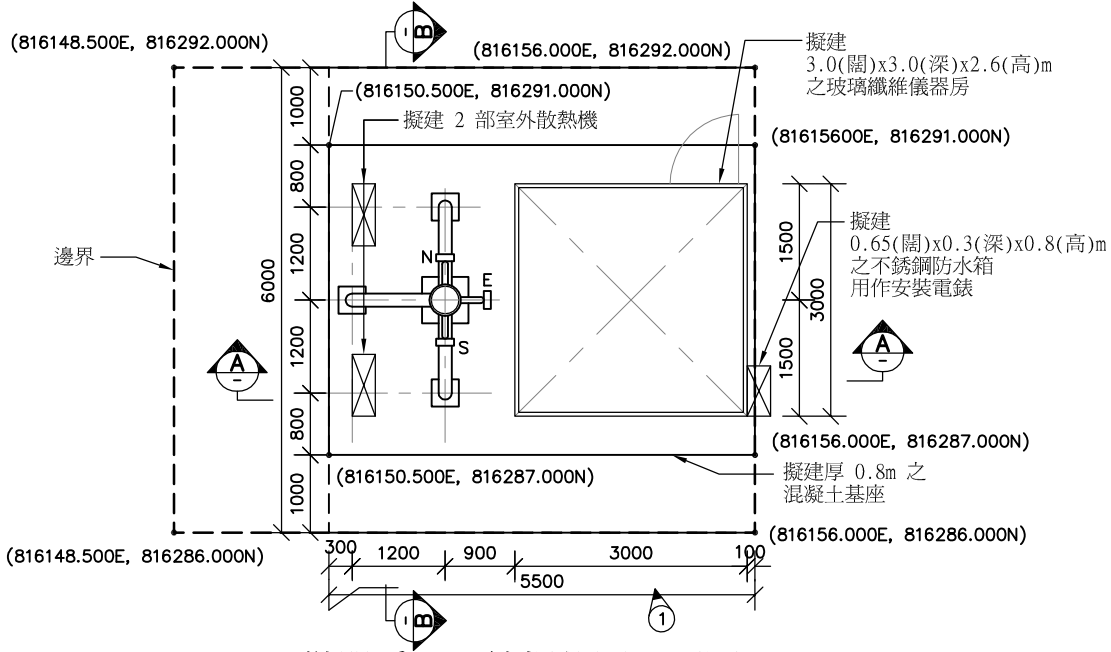
儀器房及天線桿位置平面圖
