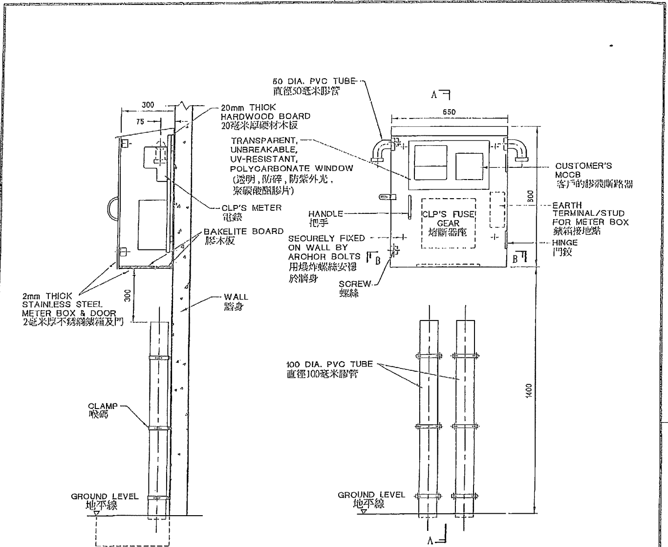
正視圖
