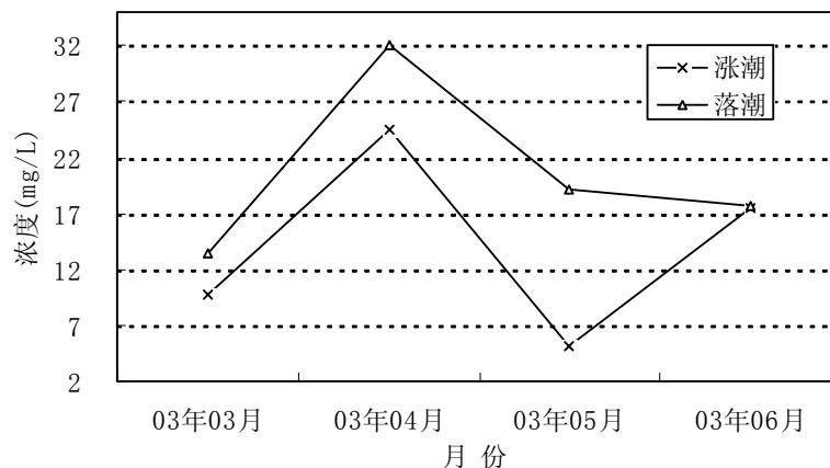
图5-6 深圳河鹿丹村站(M1) 氨氮变化趋势图
