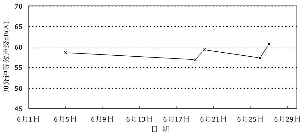
图4-3 2003年06月深圳边检宿舍昼间噪音声级变化趋势
