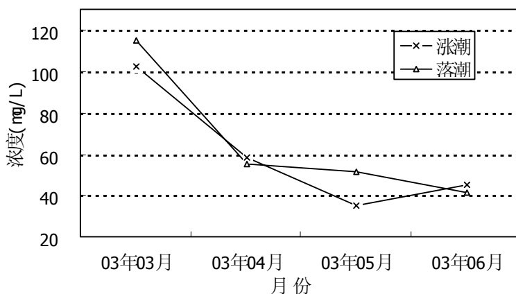
图5-3 深圳河鹿丹村站(M)SS变化趋势图
