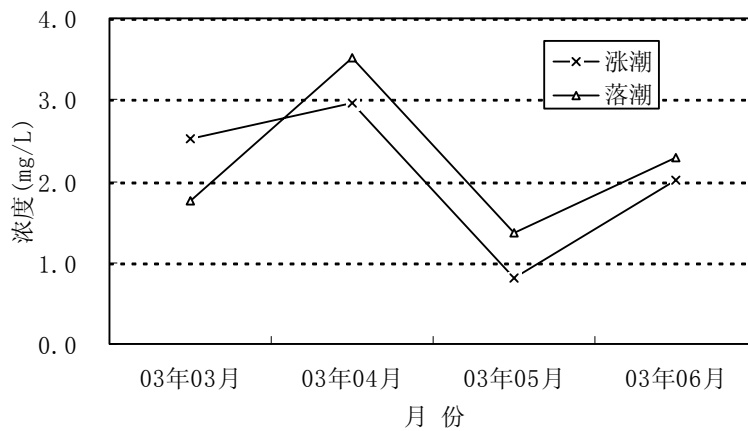
图5-8 深圳河鹿丹村站(M1)总磷变化趋势图
