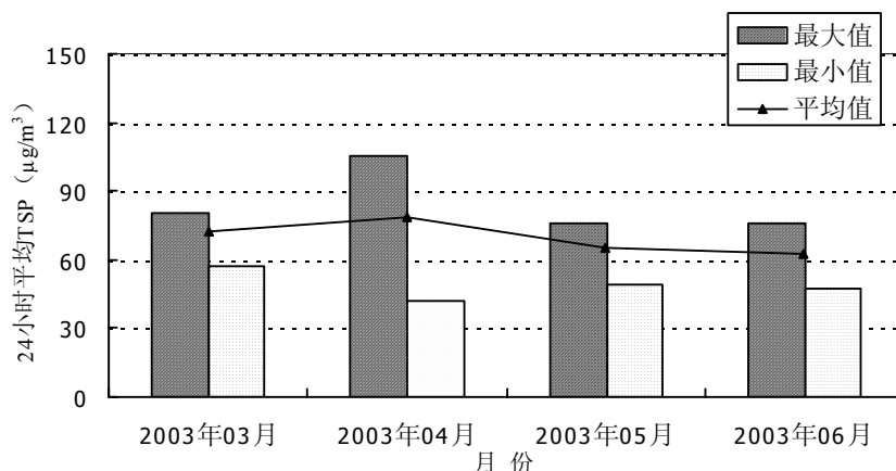
图3-5 03年03至06月边检站宿舍24小时TSP变化趋势
