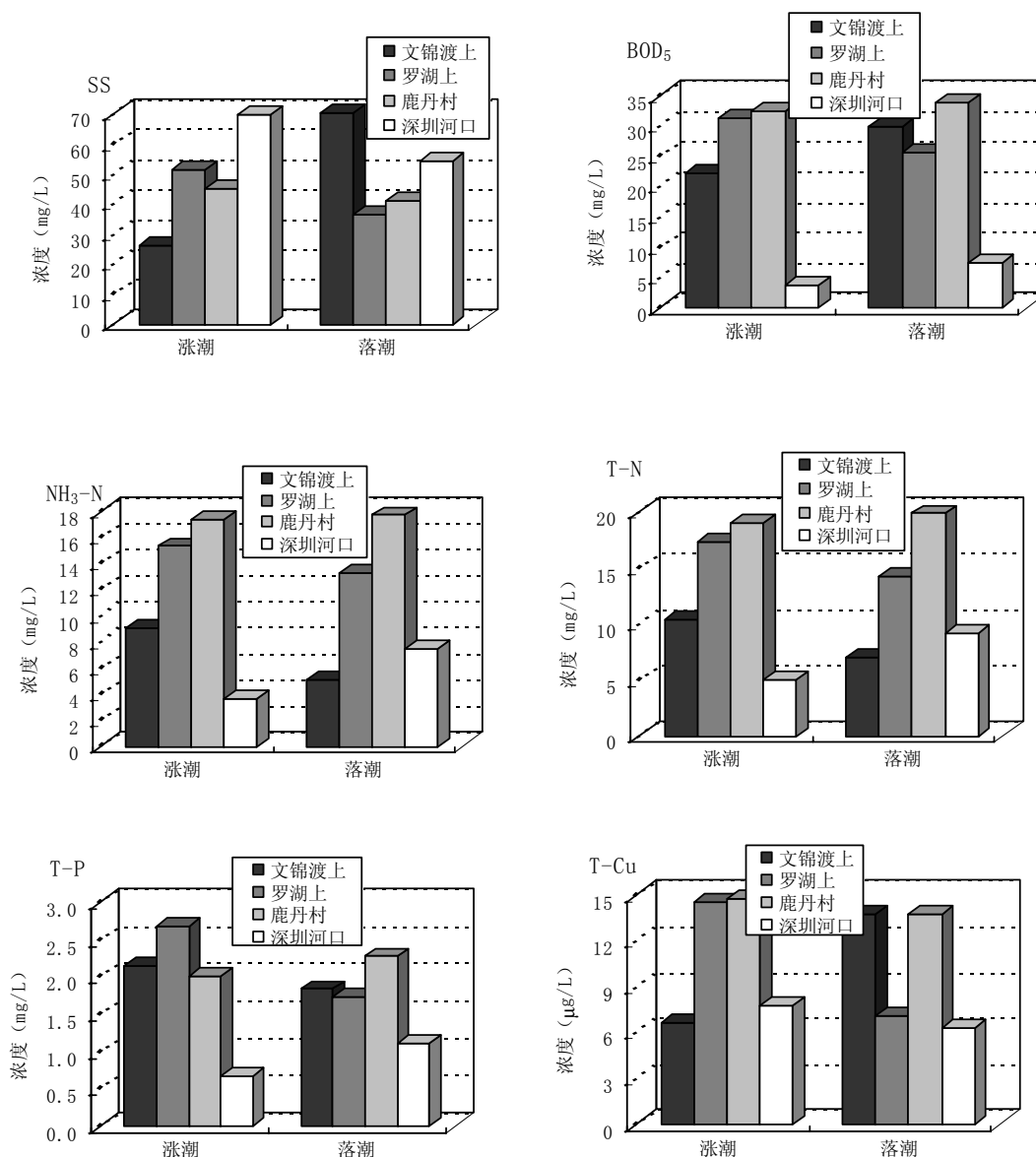
图 5-2 2003 年 6 月 3 日深圳河水水质沿程变化图
