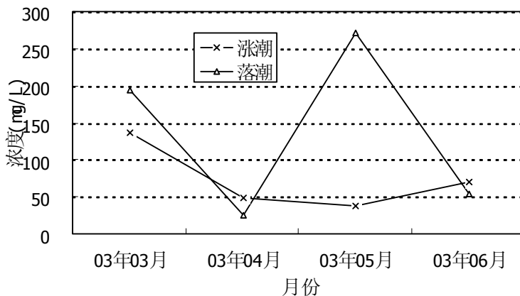
图5-4 深圳河河口站(MI)SS变化趋势图
