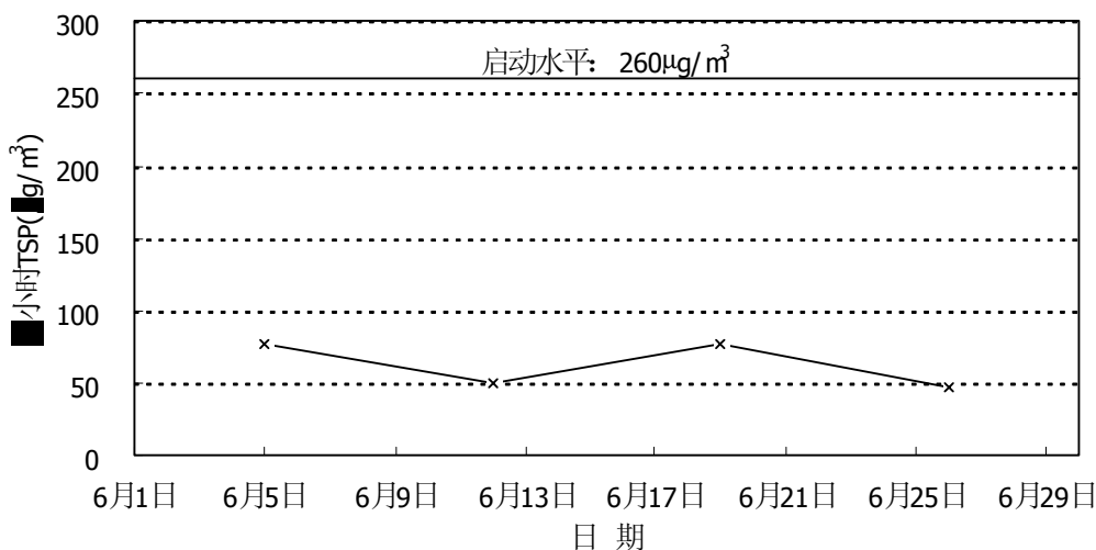
图3-3 2003年06月深圳边检宿舍24小时平均TSP变化趋势
