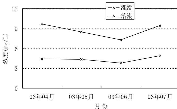
图5-10 深圳河河口站(MII) BOD 5 变化趋势图
