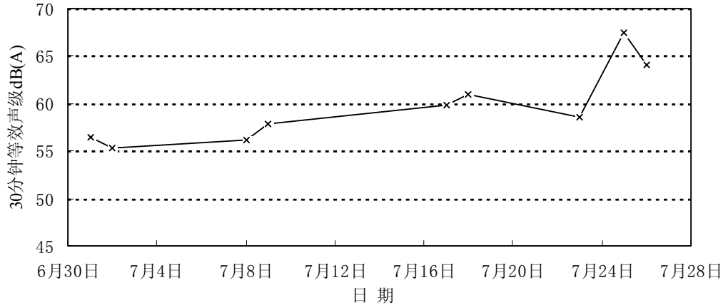
图4-3 2003年07月深圳边检宿舍昼间噪音声级变化趋势
