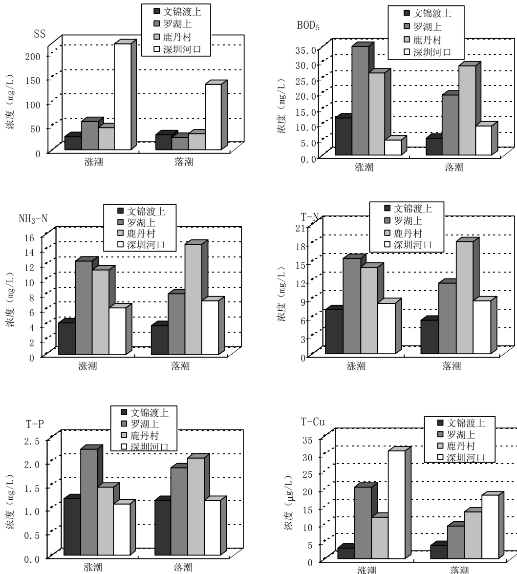
图 5-2 2003 年 7 月 3 日深圳河水水质沿程变化图
