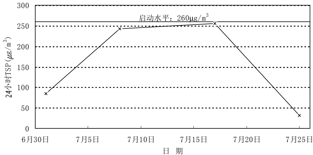
图3-2 2003年07月深圳罗湖四村24小时平均TSP变化趋势
