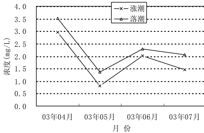
图5-8 深圳河鹿丹村站(M1) 总磷变化趋势图
