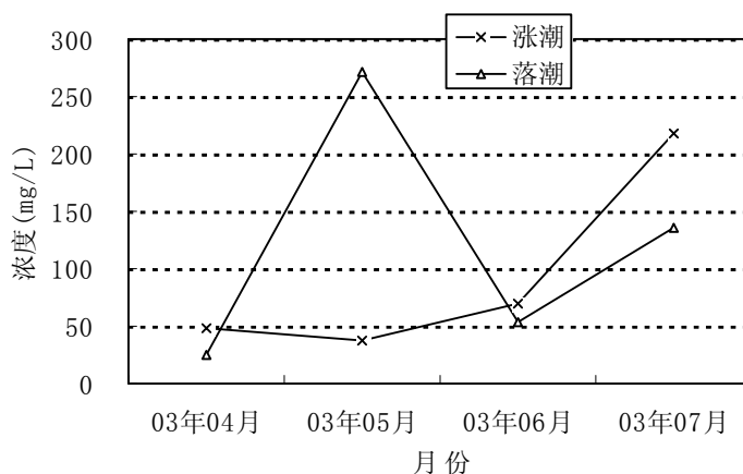
图5-4 深圳河河口站(M11)SS变化趋势图
