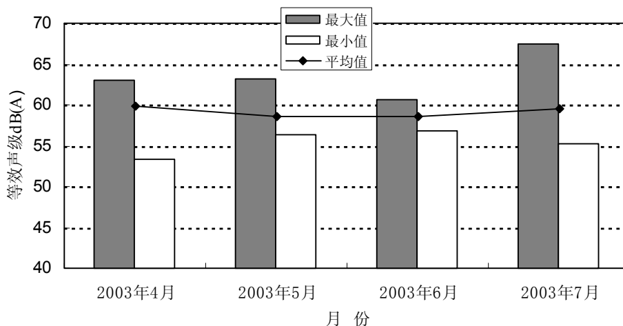
图4-5 深圳边检宿舍2003年04月~07月昼间噪音变化趋势
