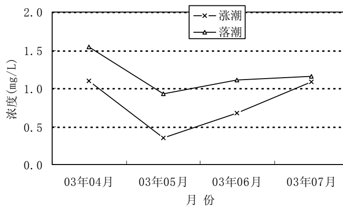
图5-13 深圳河河口站(M11)总磷变化趋势图
