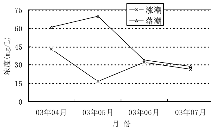
图5-5 深圳河鹿丹村站(M1)BOD 5 变化趋势图
