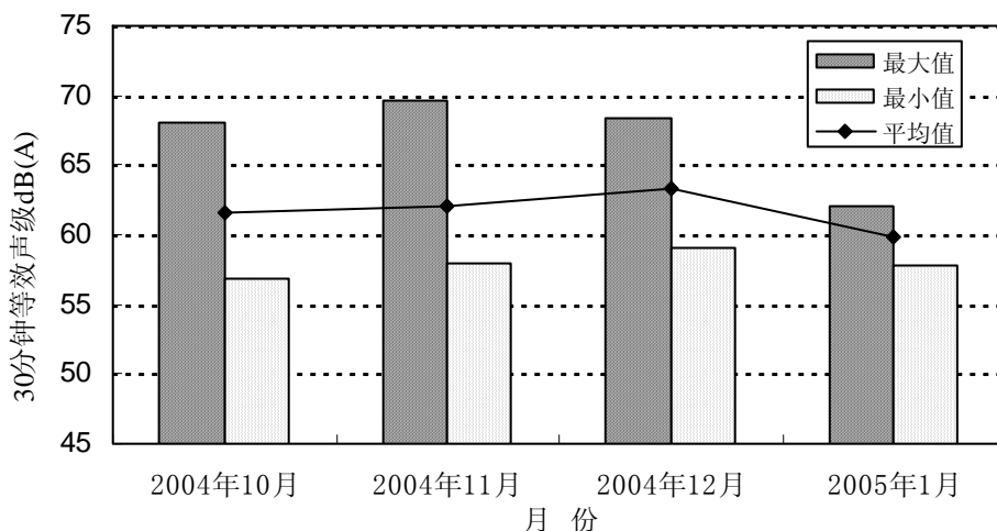
图4-4 罗湖四村05年10月~05年01月昼间噪音变化趋势
