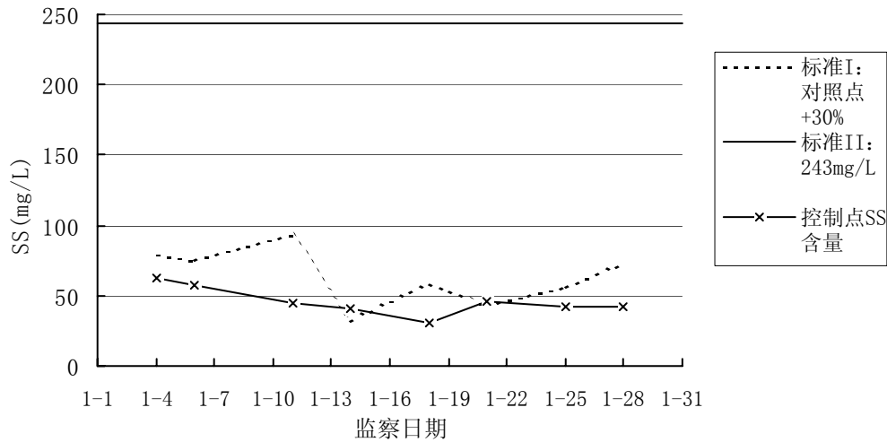
图5-3 III B工程2005年1月落潮期修坡施工SS含量超标情况对照图
