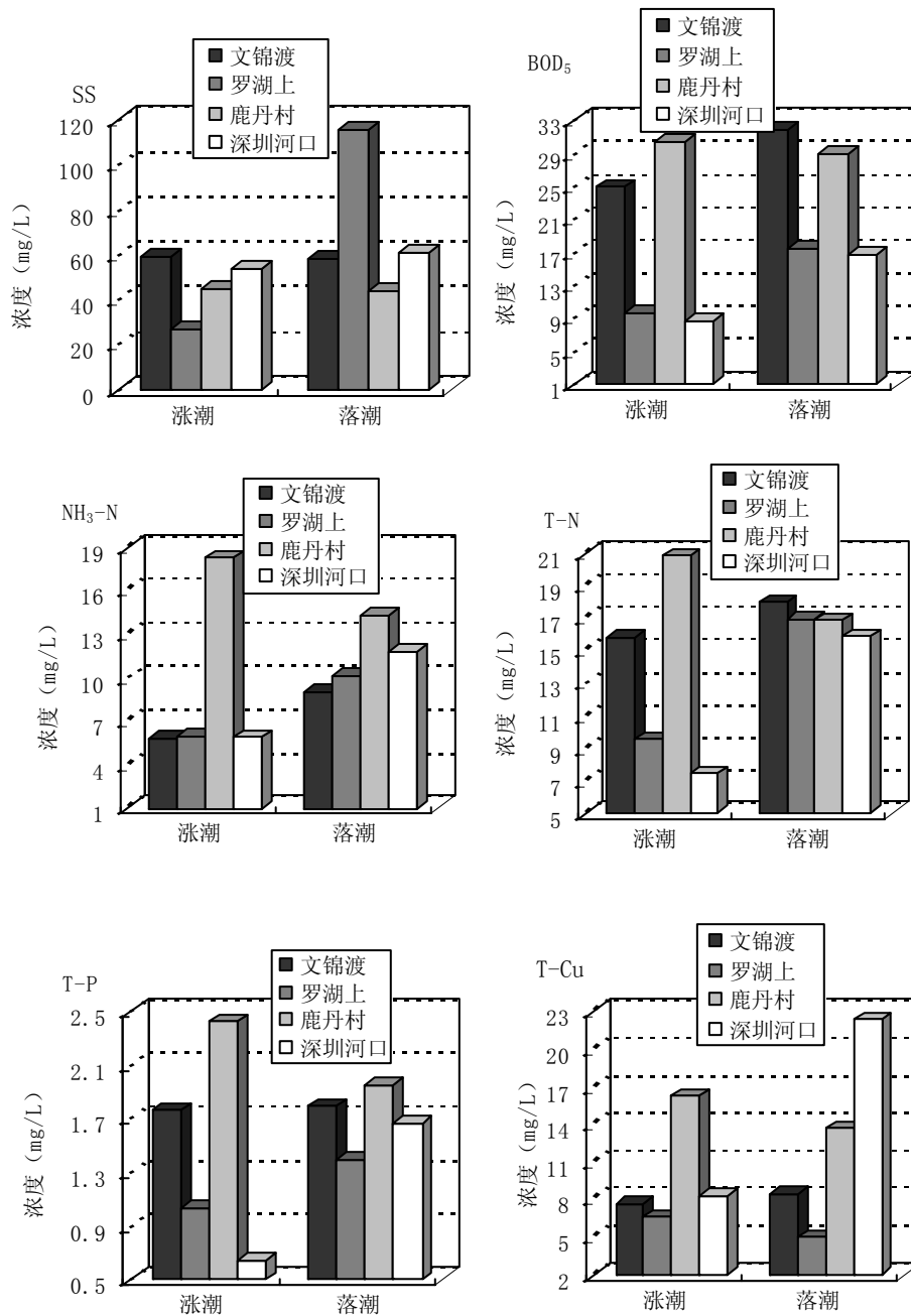
图 5-4 2005 年 1 月 6 日深圳河水质沿程变化图
