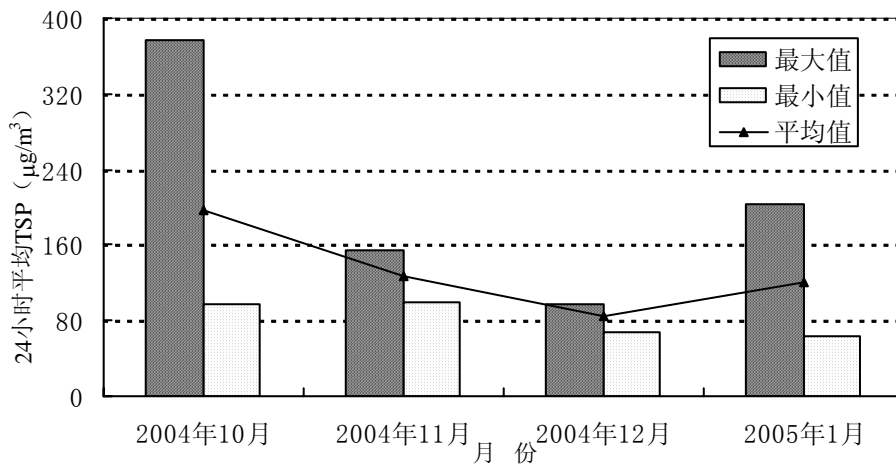
图3-4 04年10月至05年1月深圳罗湖四村24小时TSP变化趋势
