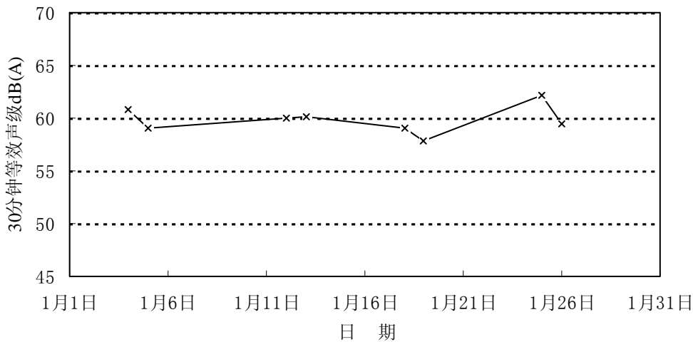
图4-2 2005年1月罗湖四村昼间噪音声级变化趋势
