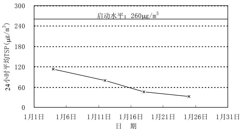
图3-3 2005年1月深圳边检宿舍24小时平均TSP变化趋势
