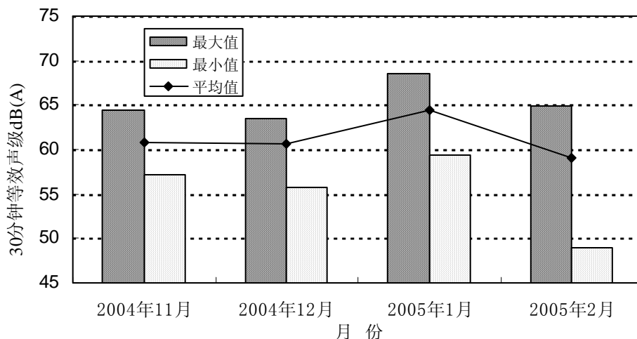
图4-5 华侨新村04年11月~05年02月昼间噪音变化趋势
