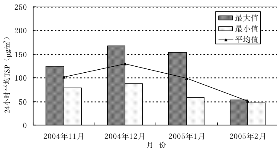
图3-6 04年11月至05年2月香港瓦窑村24小时TSP变化趋势
