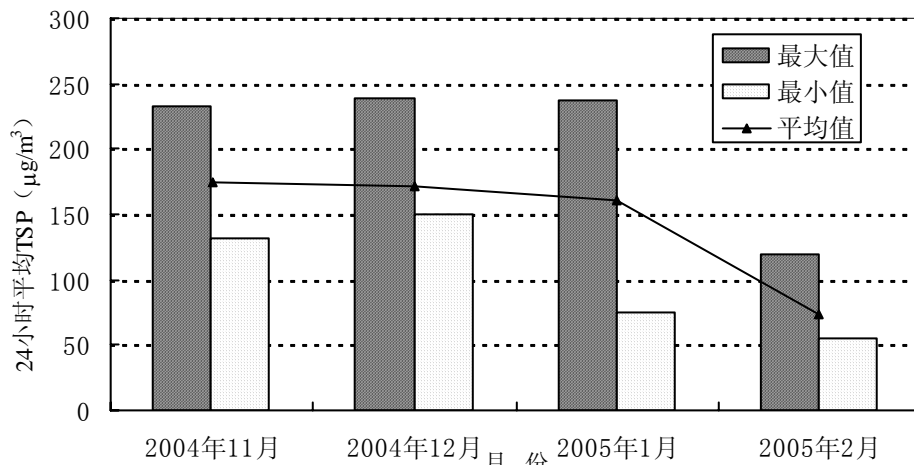
图3-5 04年11月至05年2月深圳华侨新村24小时TSP变化趋势
