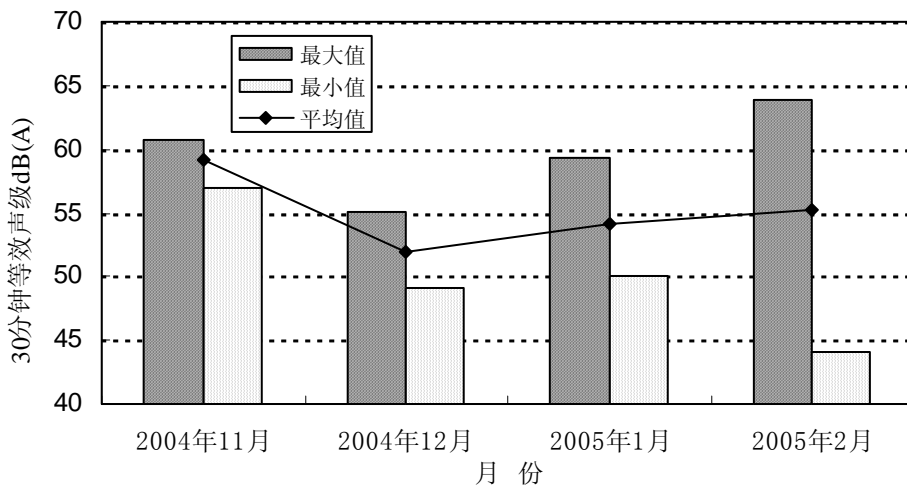
图4-7 香港木湖村04年11月~05年02月昼间噪音变化趋势
