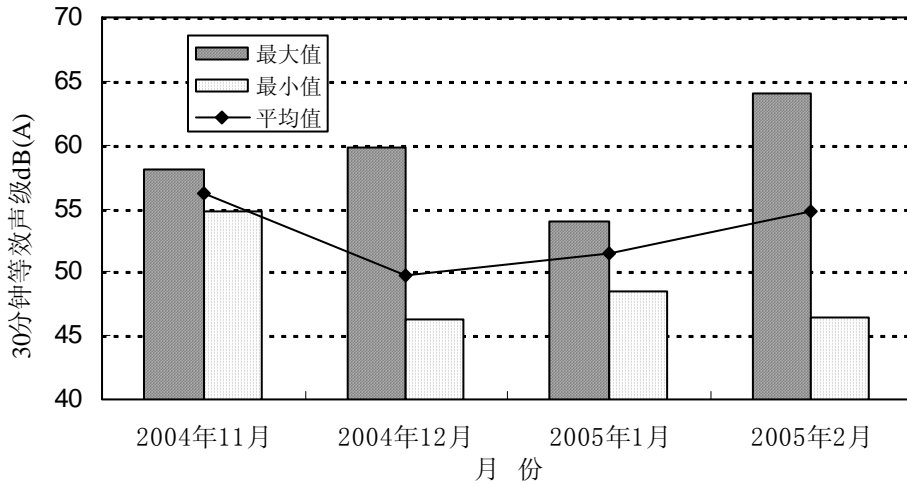
图4-6 香港瓦窑村04年11月~05年02月昼间噪音变化趋势
