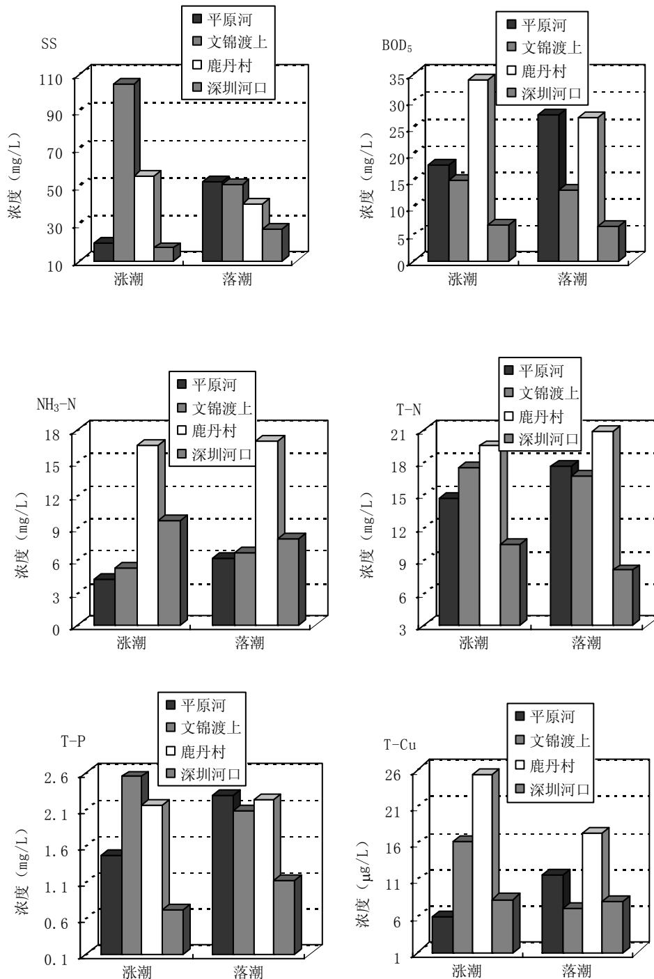
图 5-2 2005 年 2 月 16 日深圳河水水质沿程变化图
