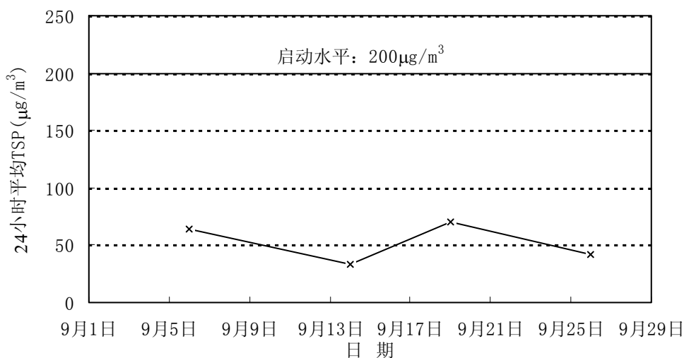
图3-4 2006年9月木湖村监察点24小时平均TSP变化趋势
