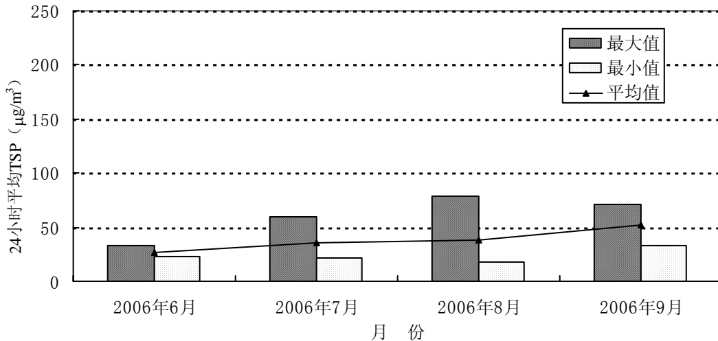
图3-7 2006年6月至9月香港木湖村监察点24小时TSP变化趋势
