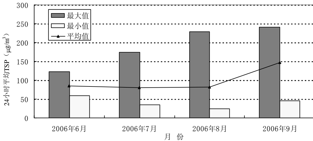
图3-5 2006年6月至9月华侨新村监察点24小时TSP变化趋势
