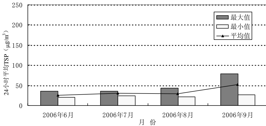
图3-6 2006年6月至9月香港瓦窑村监察点24小时TSP变化趋势
