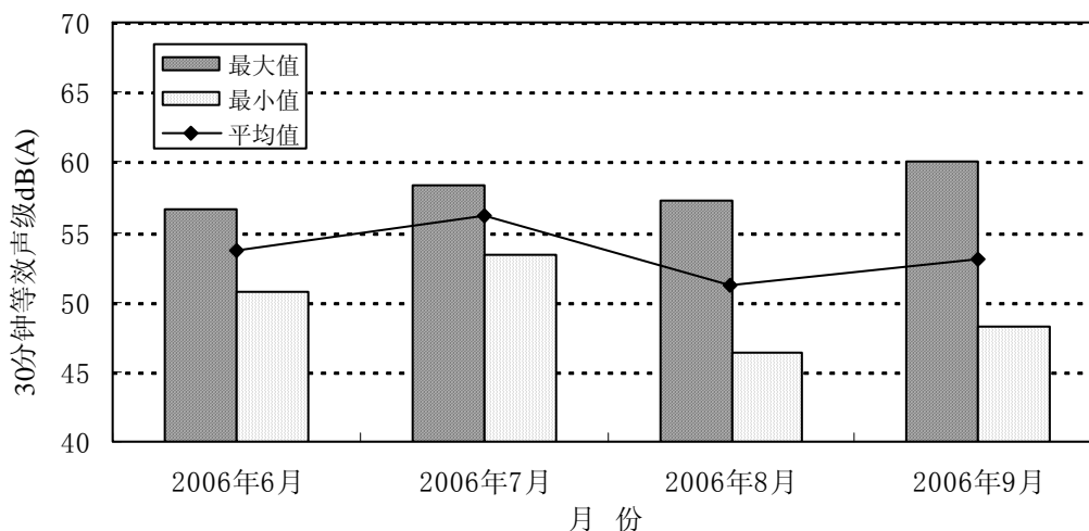
图4-6 2006年6月~9月瓦窑村监察点昼间噪音变化趋势
