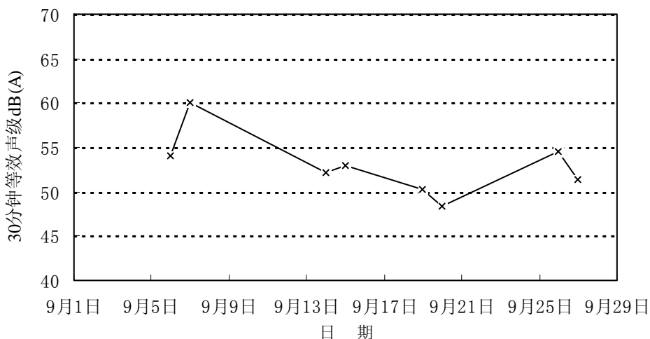
图4-3 2006年9月瓦窑村监察点昼间噪音声级变化趋势
