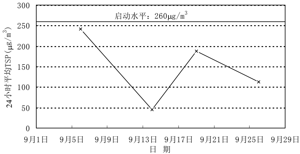
图3-2 2006年9月华侨新村监察点24小时平均TSP变化趋势
