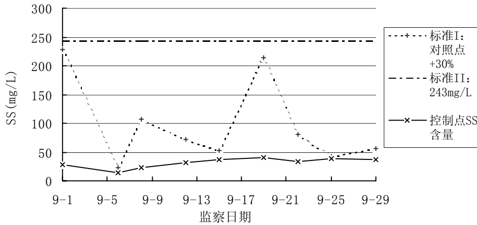
图5-5 2006年09月III C工程落潮期水下疏浚SS含量超标情况对照图
