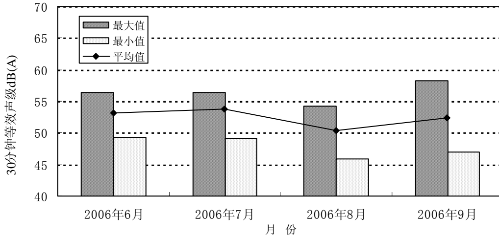
图4-7 2006年6月~9月木湖村监察点昼间噪音变化趋势
