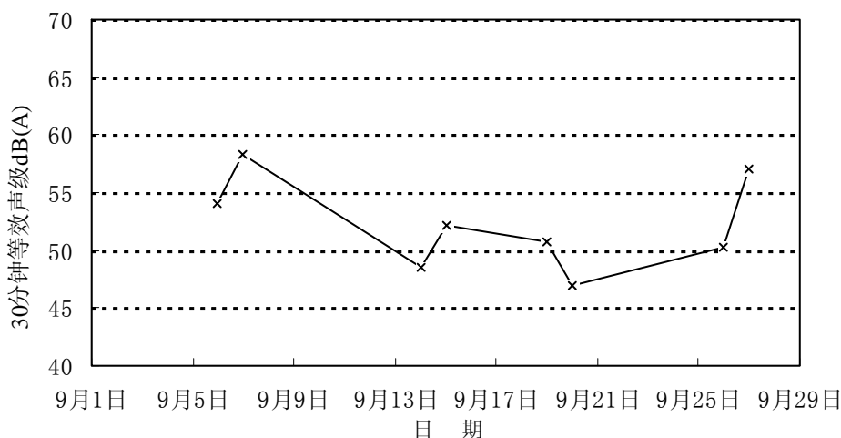
图4-4 2006年9月木湖村监察点昼间噪音声级变化趋势
