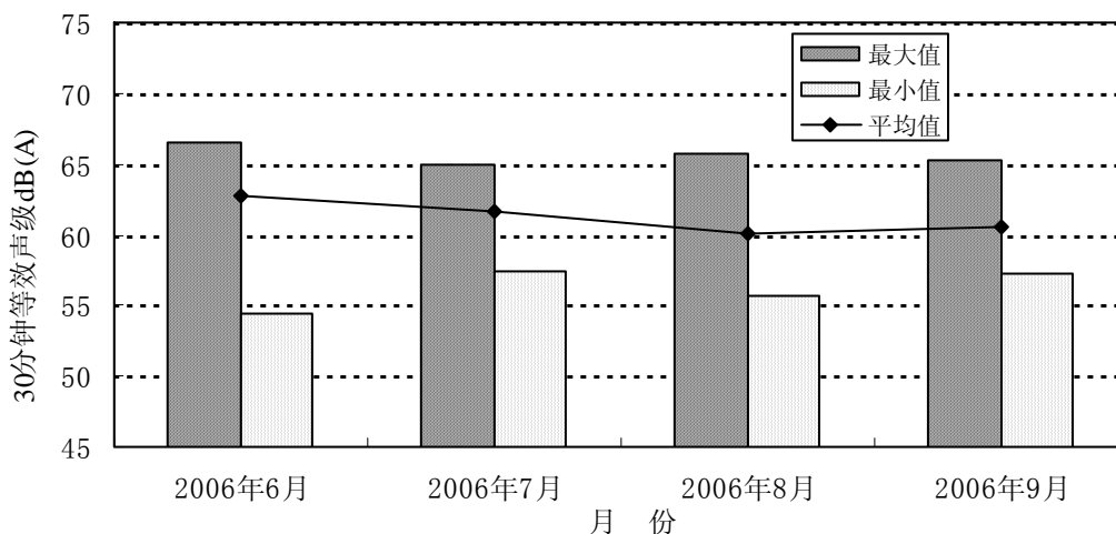
图4-5 2006年6月~9月华侨新村监察点昼间噪音变化趋势
