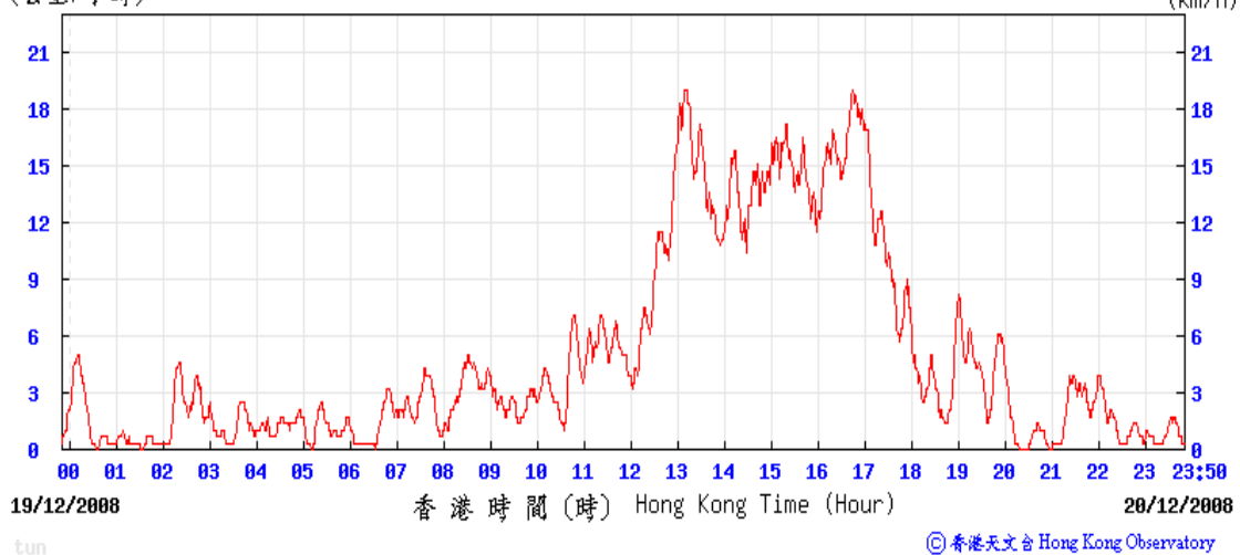
(公里/小時) (於香港時間 2008 年12月20日23時50分更新) (Updated at 23:50H on 20 Dec 2008) (km/h)
