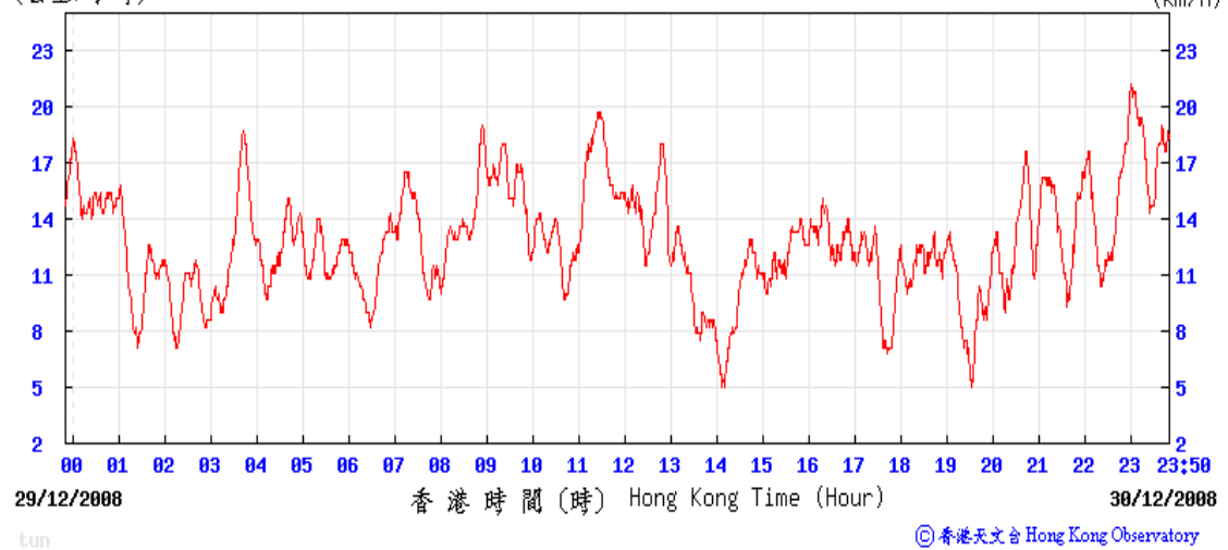
(公里/小時) (於香港時間 2008 年12月30日23時50分更新) (Updated at 23:50H on 30 Dec 2008) (km/h)
