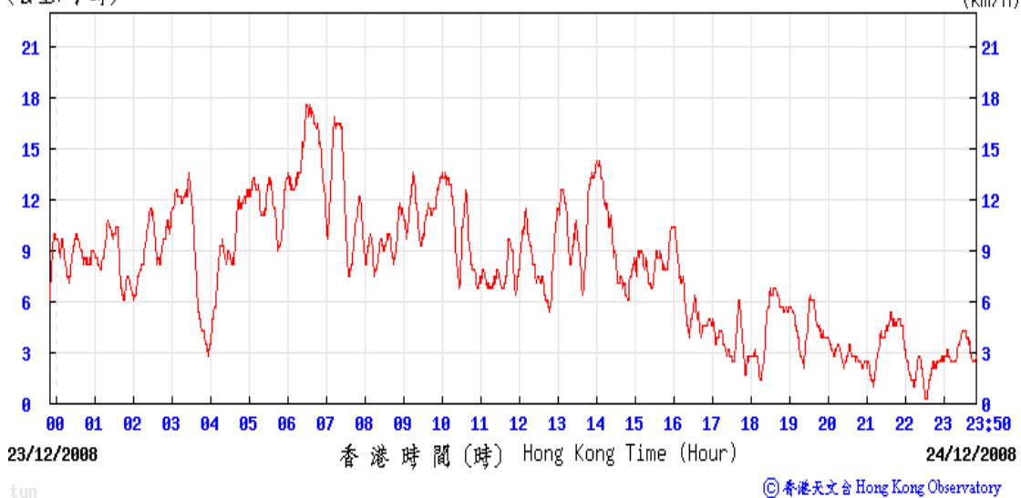
(公里/小時) (於香港時間 2008 年12月24日23時50分更新) (Updated at 23:50H on 24 Dec 2008) (km/h)
