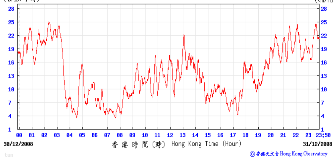
(公里/小時) (於香港時間 2008 年12月31日23時50分更新) (Updated at 23:50H on 31 Dec 2008) (km/h)
