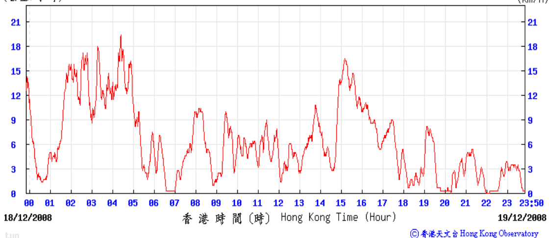
(公里/小時) (於香港時間 2008 年12月19日23時50分更新) (Updated at 23:50H on 19 Dec 2008) (km/h)
