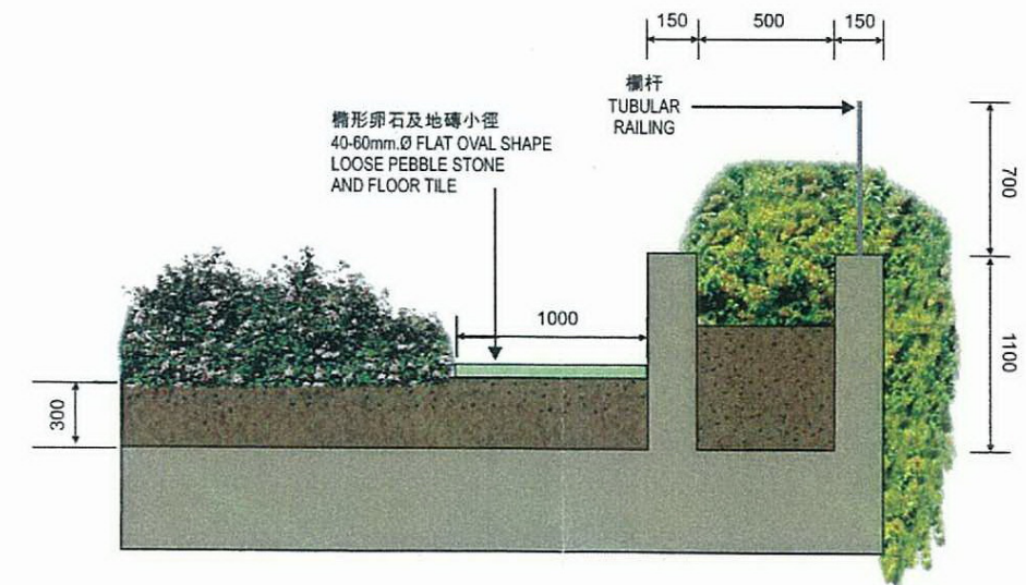
切面A-A SECTION A-A
