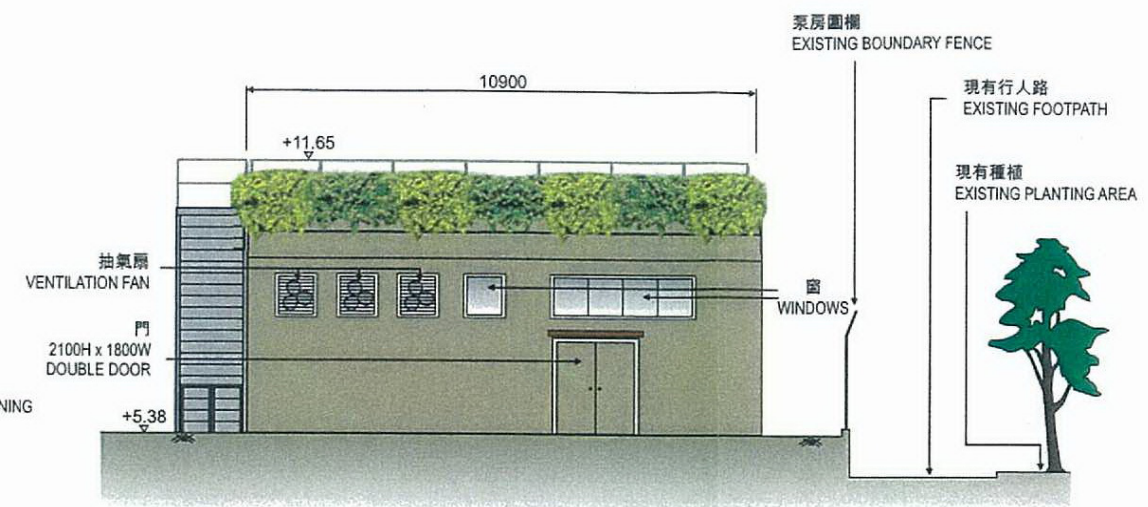
西面立視圖 WESTERN ELEVATION
