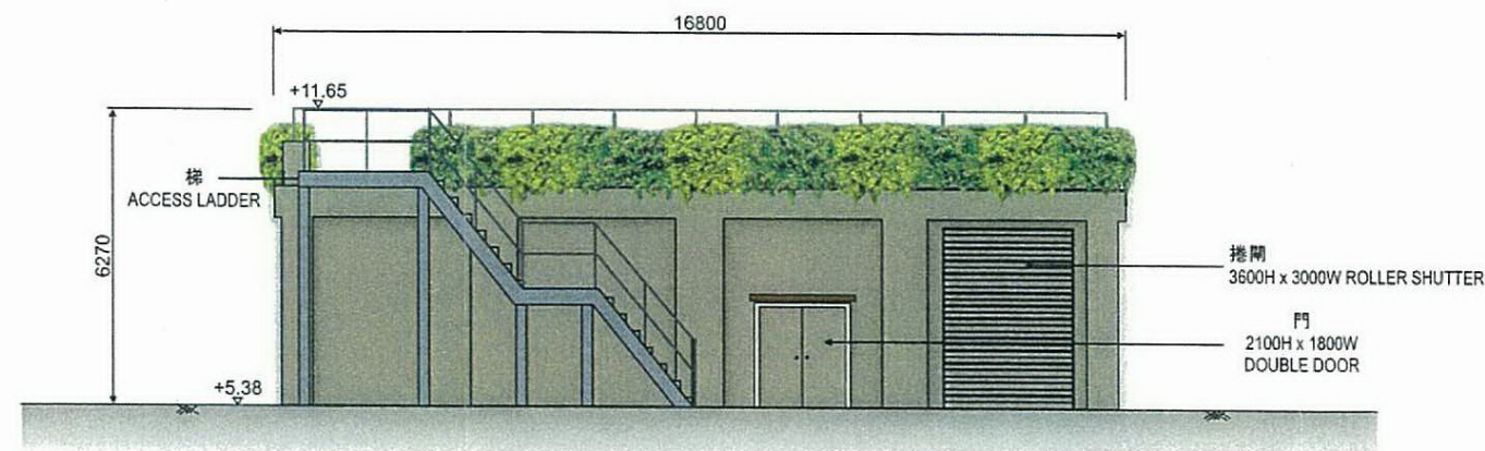
北面立視圖 NORTHERN ELEVATION
