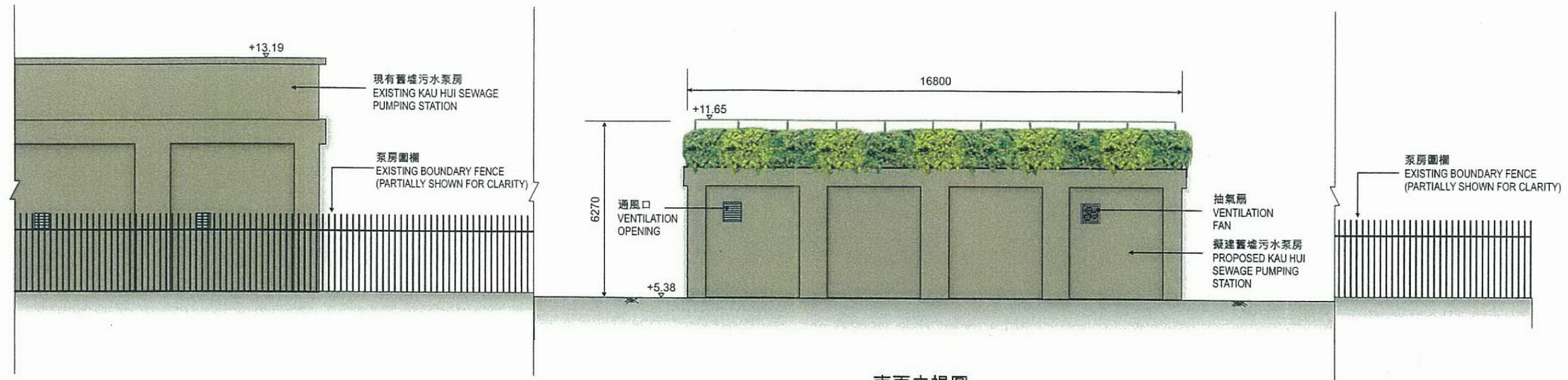
南面立視圖 SOUTHERN ELEVATION
