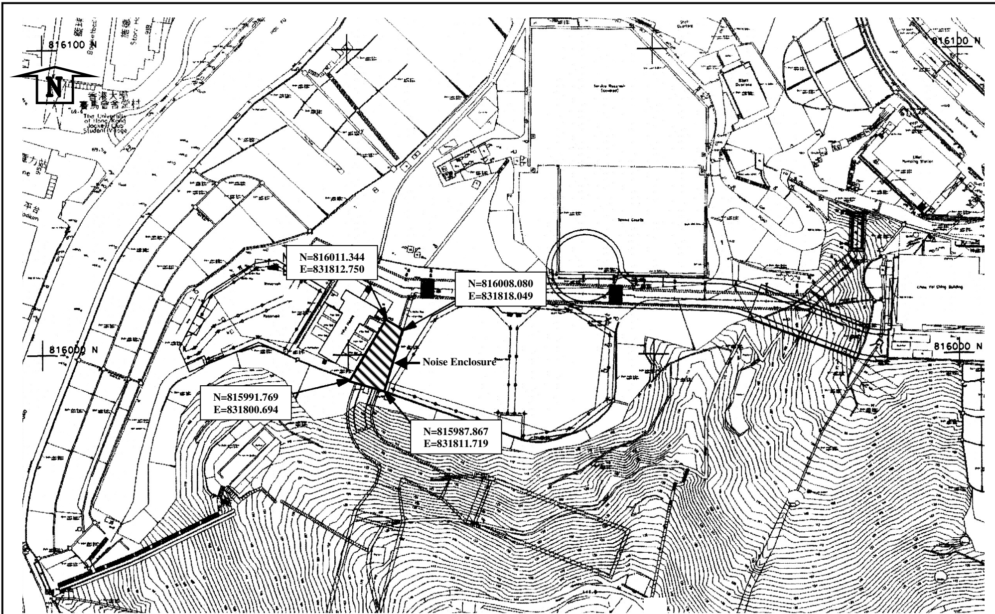
Figure 3a : Noise Enclosure Design Plan - Location Plan of Noise Enclosure 圖 3a : 隔音罩設計圖 - 隔音罩位置
