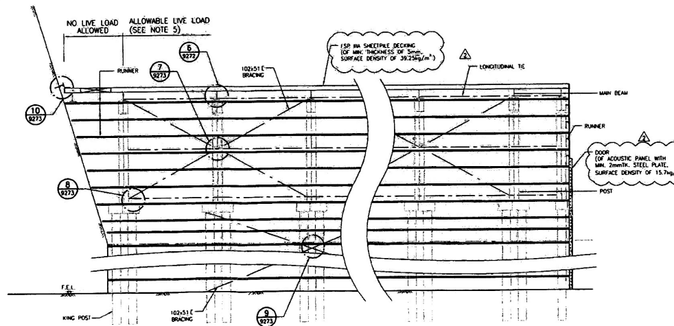
Section C - C 切面圖 C - C
