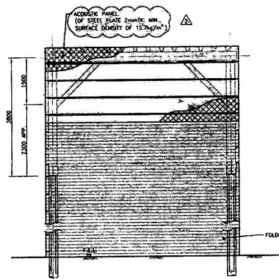
Section B - B 切面圖 B - B
