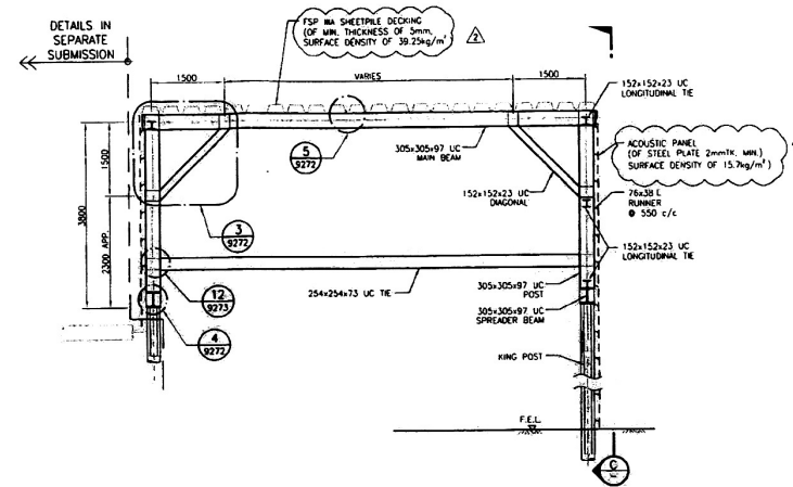
Section A - A 切面圖 A - A
