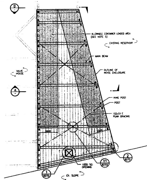
Framing Plan 構架圖
