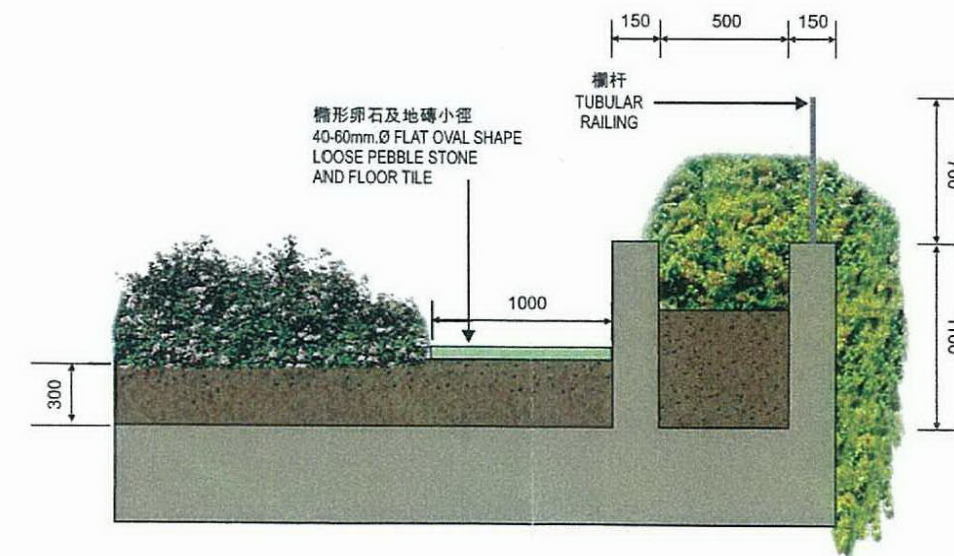
切面A-A SECTION A-A
