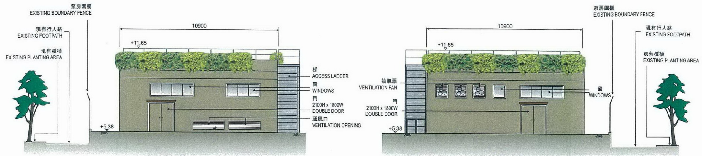
東面立視圖 EASTERN ELEVATION
