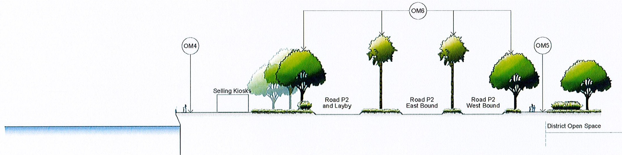
Section A-A
