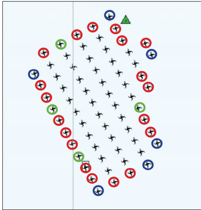
3MW LAYOUT
