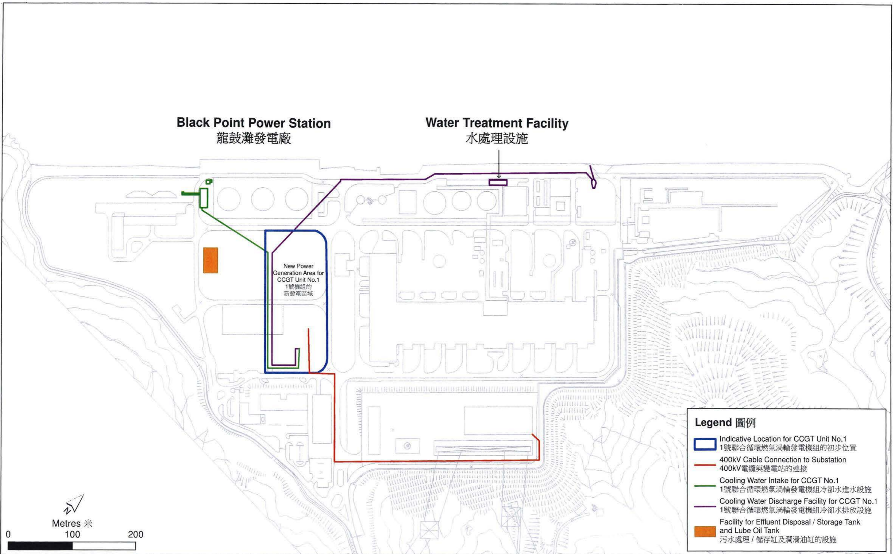
Figure 1 圖 1 Additional Gas-fired Generation Units Project - Indicative Location Plan of Key Project Components for CCGT Unit No.1 新增燃氣發電機組工程 - 1號聯合循環燃氣渦輪發電機組主要工程項目組成部份的初步位置圖
