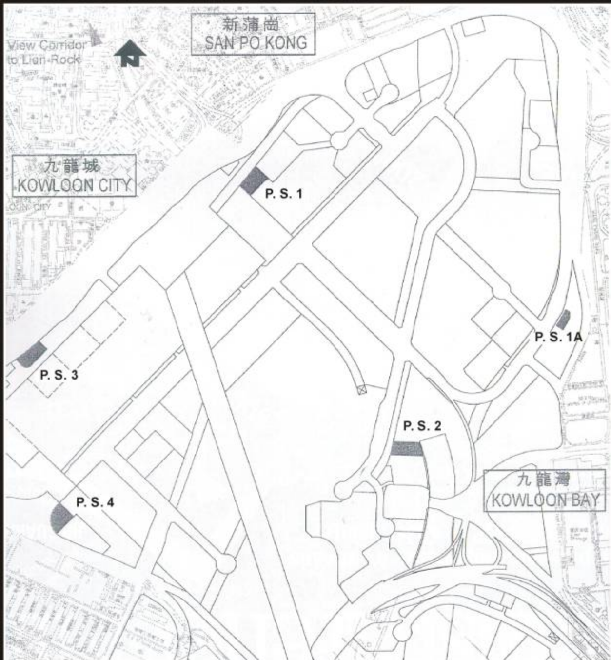
擬建污水泵站位置圖
