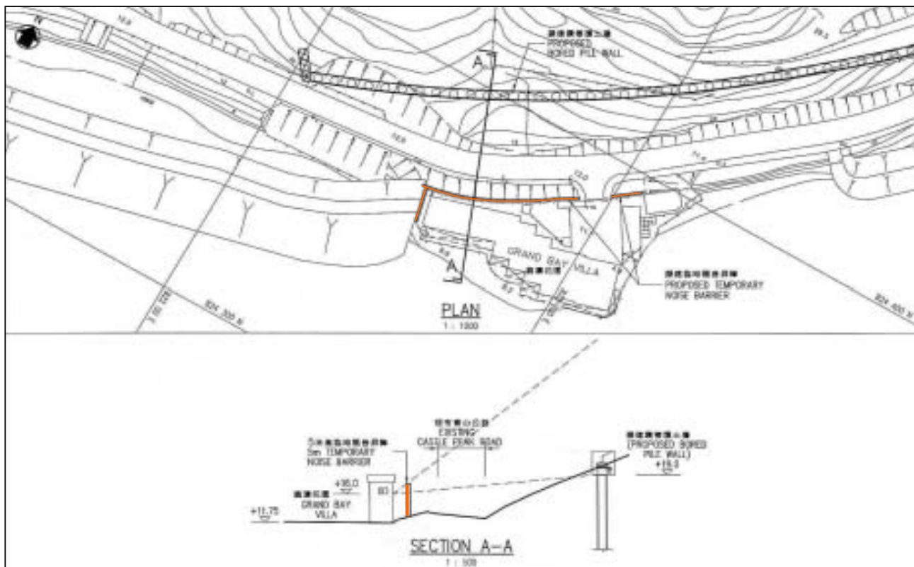
荃灣第二區與嘉龍村之間的青山公路改善工程 於龍瀟花園擬建臨時隔音屏障
