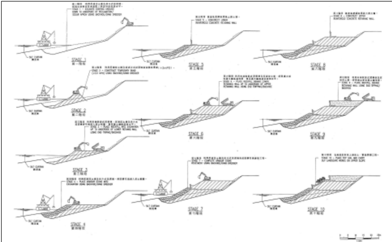
荃灣第二區與嘉龍村之間的青山公路改善工程 龍瀟花園以西填海區的建設方法
