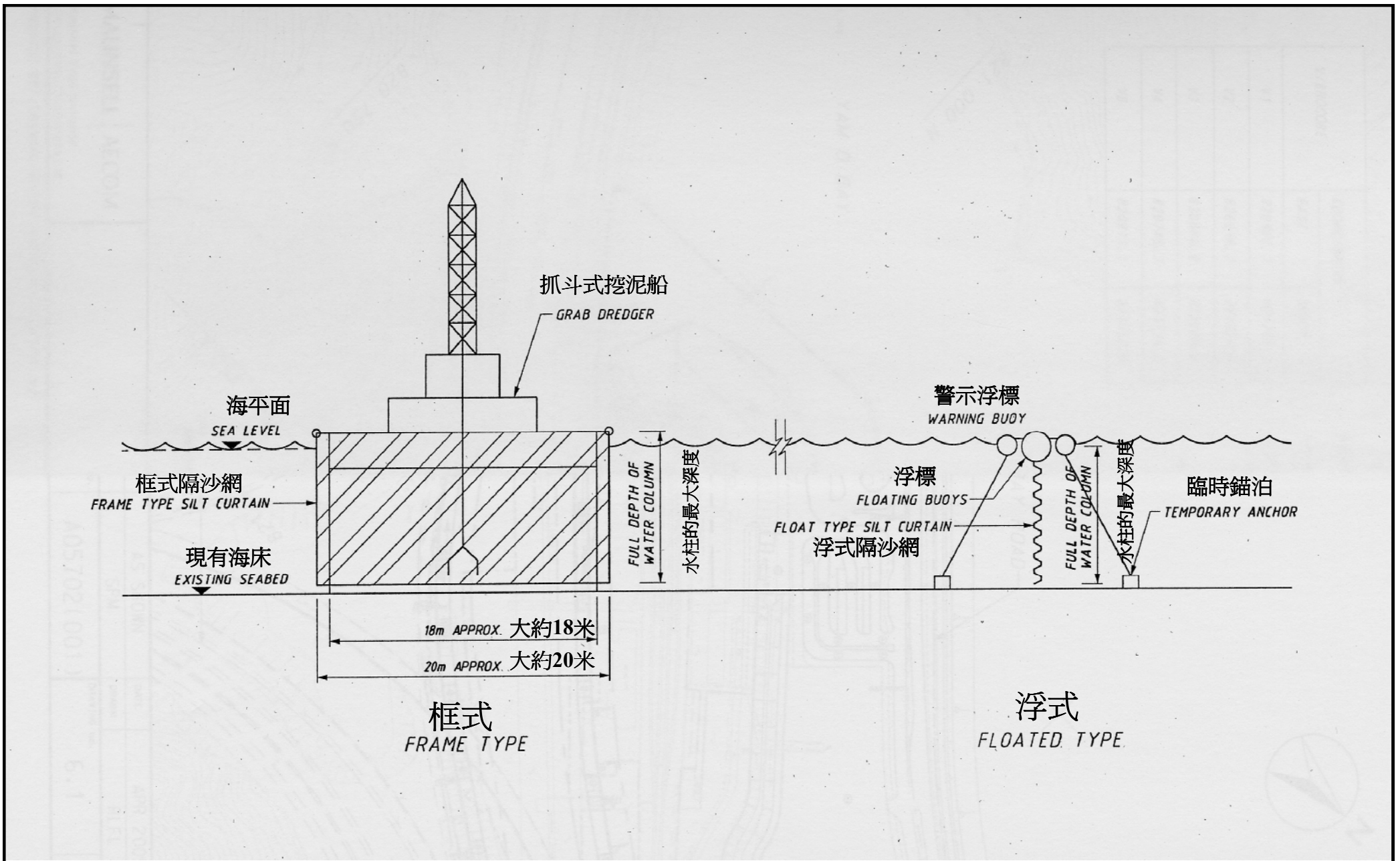
Figure 3 Sectional Configuration of Silt Curtain 圖 3 隔沙網的截面構造
