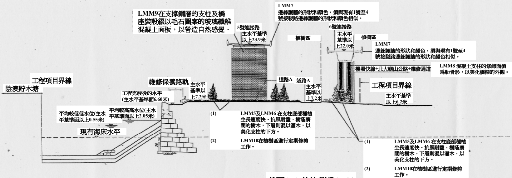
截面A-A 的比例為1:500
