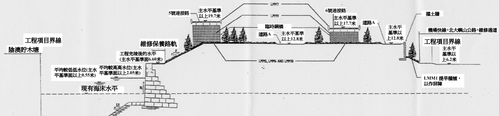
截面B-B 的比例為1:500
