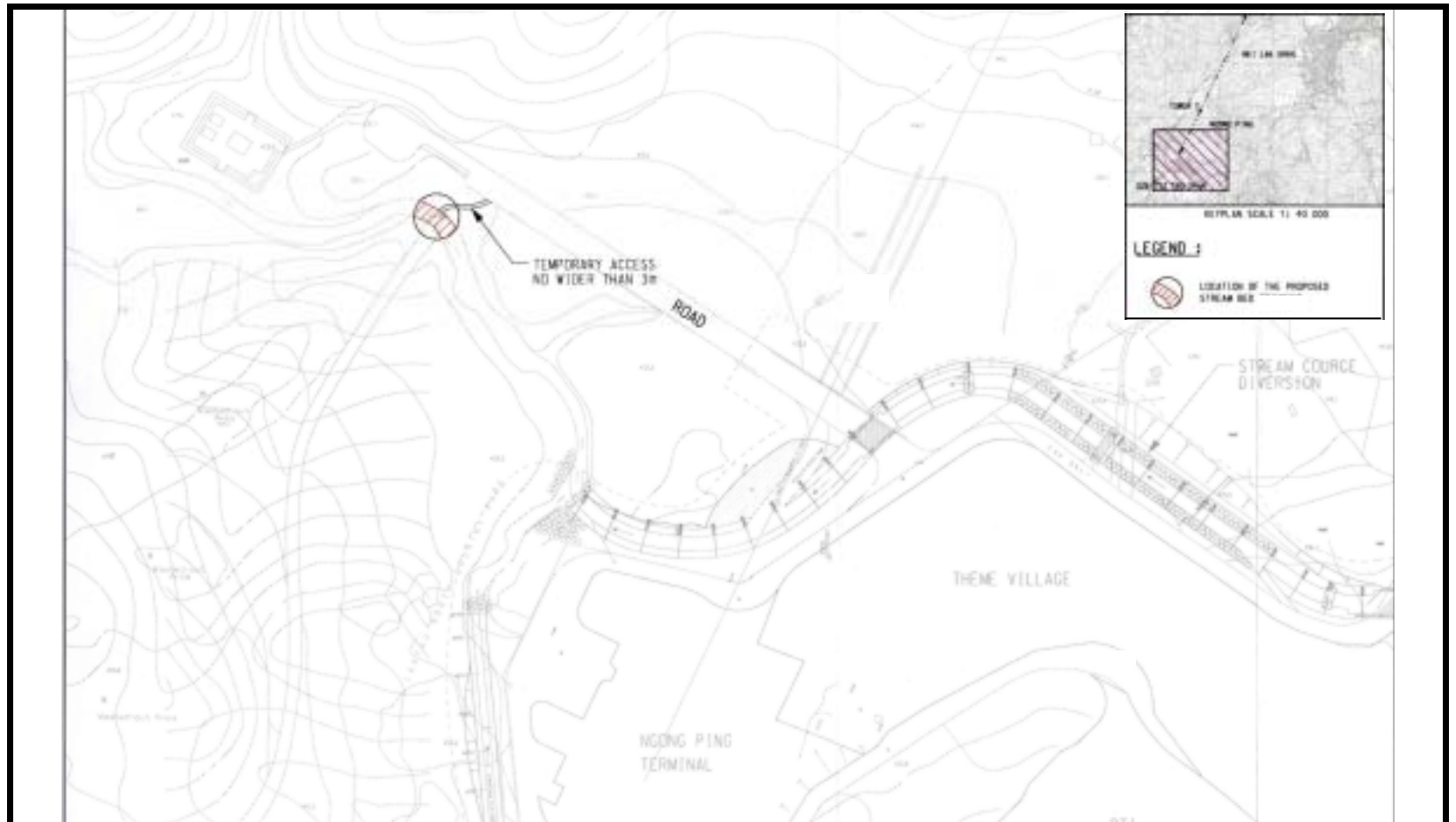
Figure 1: Location Plan of the Stream Bed Trimming at Ngong Ping 圖 1：於昂平進行溪流河床改善工程的位置圖
