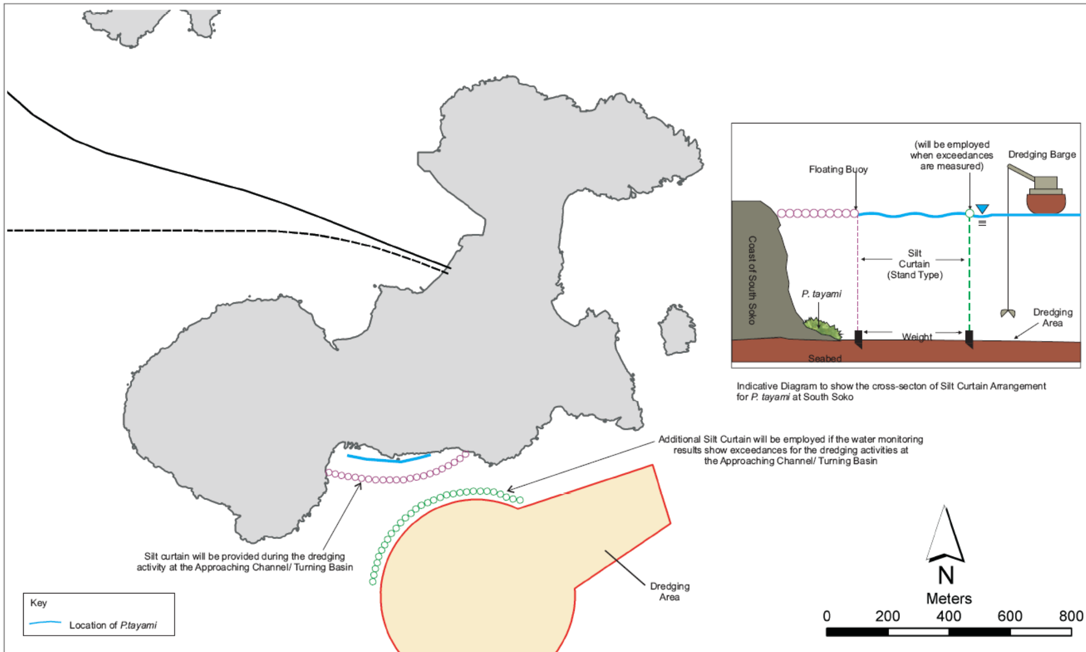
為「假鐵星珊瑚」而設的淤泥屏障〔直立式〕的安排示意圖
