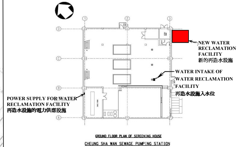
LAYOUT PLAN 平面圖 CHEUNG SHA WAN SEWAGE PUMPING STATION 長沙灣污水泵房
