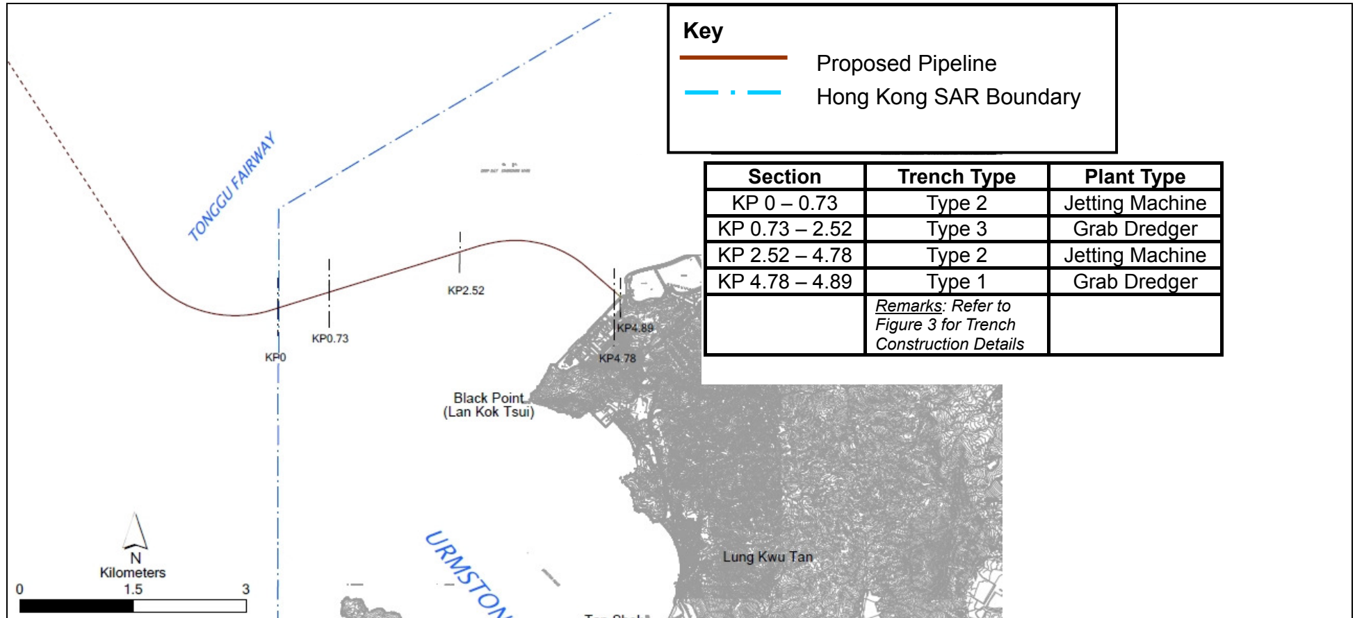
Figure 2 Black Point Gas Supply Project (Phase 1) 龍鼓灘燃氣供應項目（第一期） 圖二 Sections of the Submarine Gas Pipeline 海底輸氣管道的分段圖
