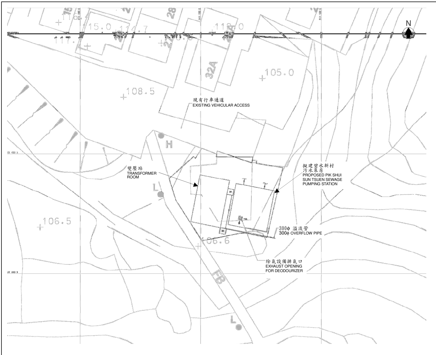
Project Title: Sewerage Works at Pik Shui Sun Tsuen 工程項目名稱：碧水新村污水收集系統工程 Pik Shui Sun Tsuen Sewage Pumping Station General Layout Plan 碧水新村污水泵房分佈圖
