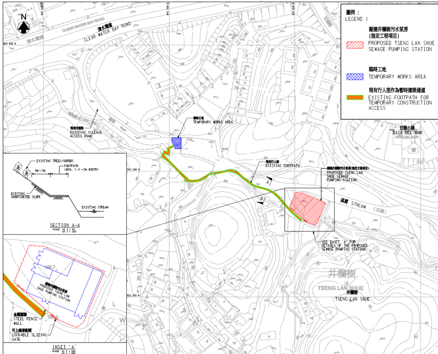
Project Title: Sewage Pumping Station at Tseng Lan Shue 工程項目名稱: 井欄樹污水泵房 Location Plan 位置圖
