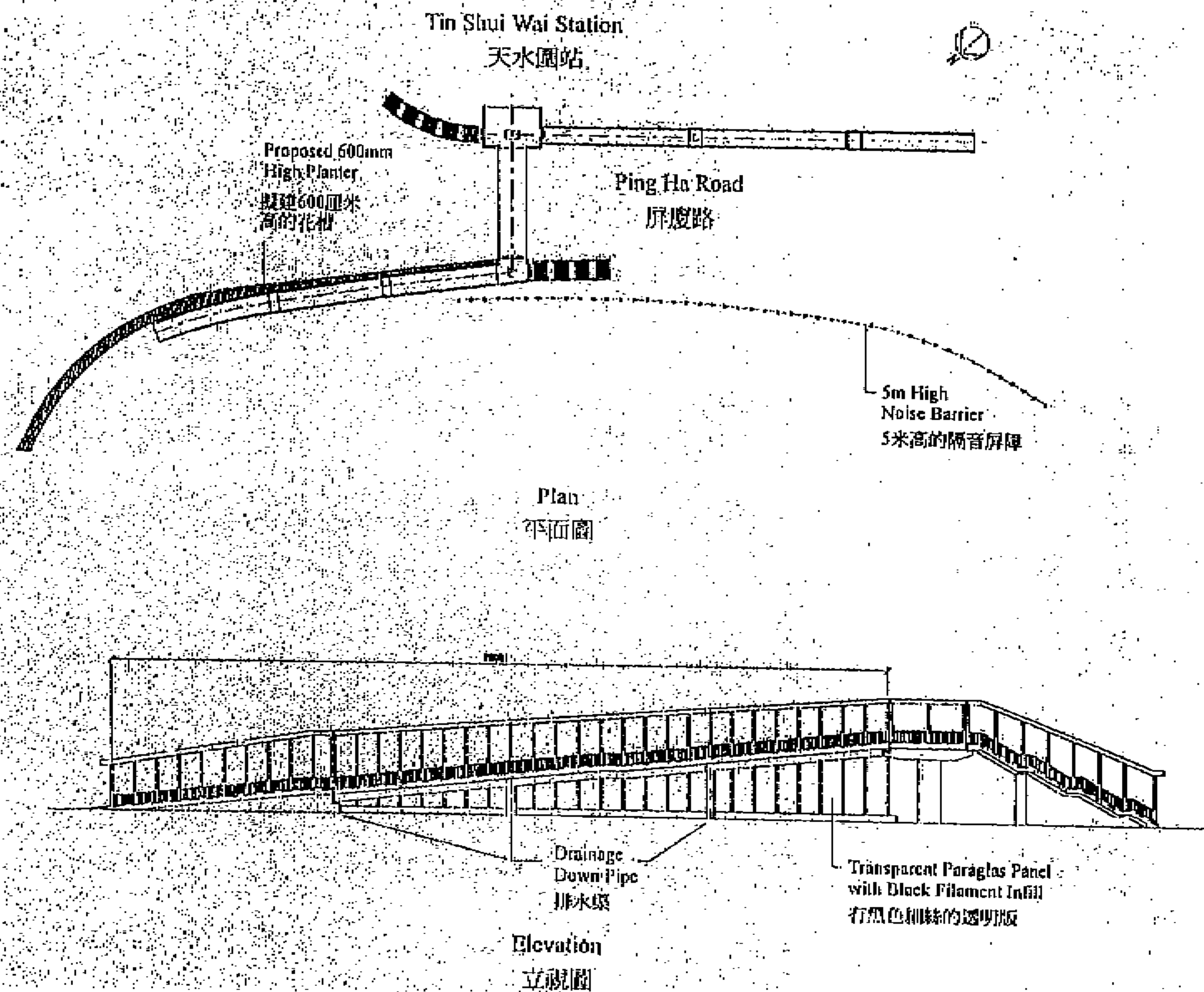
圖5.2 - 與屏廈路行人天橋連結之屏障的設計圖
