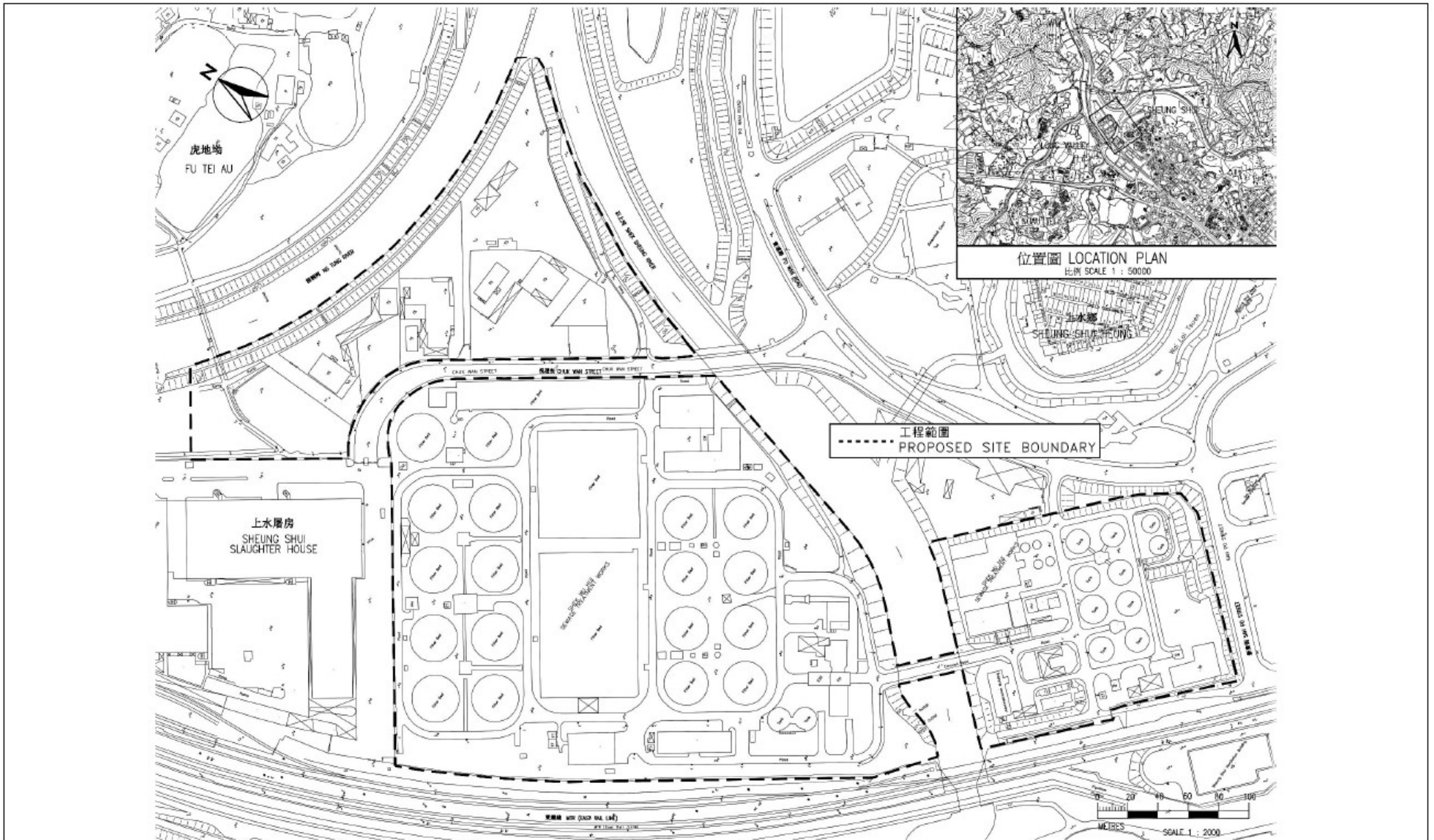
Figure 1: Location Plan 圖 1：工程位置圖
