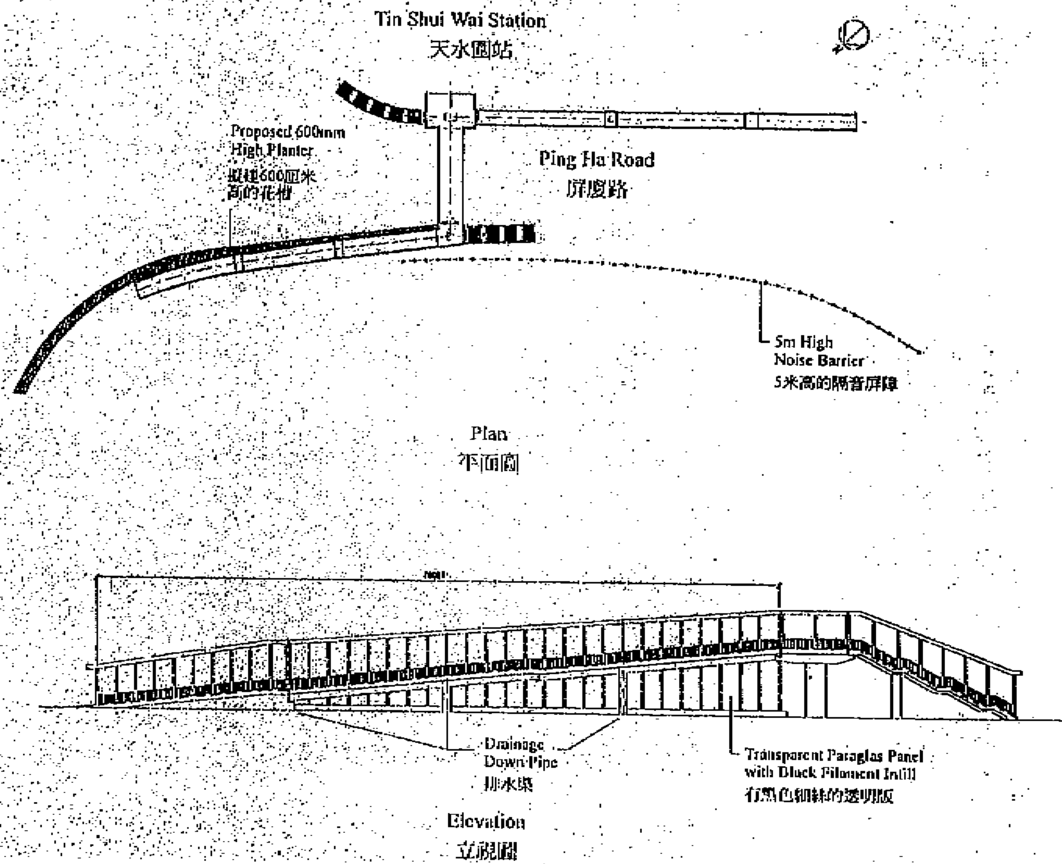
圖5.2 - 建議的與行人天橋連結之屏障的設計圖
