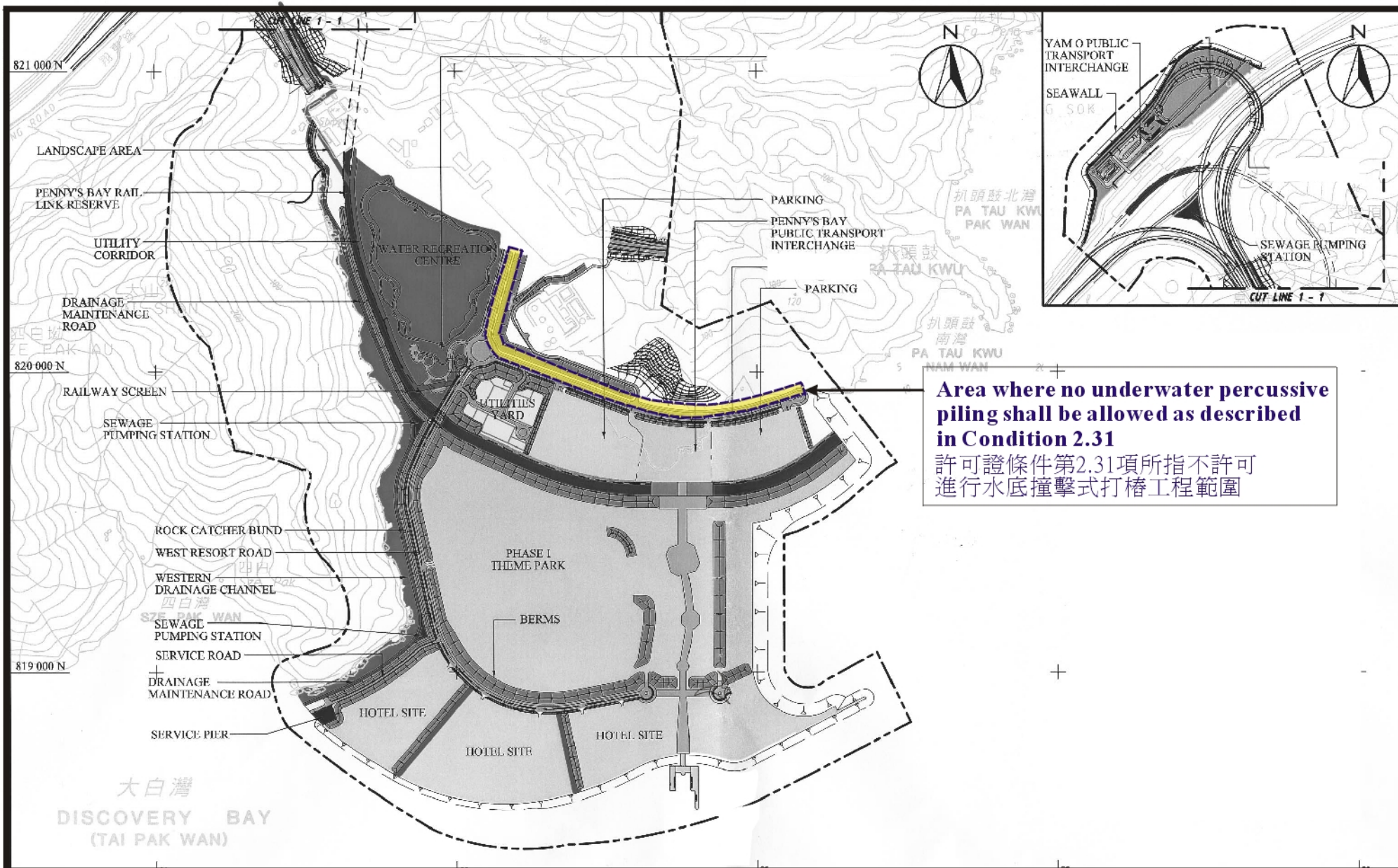
Figure 4 Restriction on Underwater Percussive Piling 圖 4 水底撞擊式打樁限制範圍
