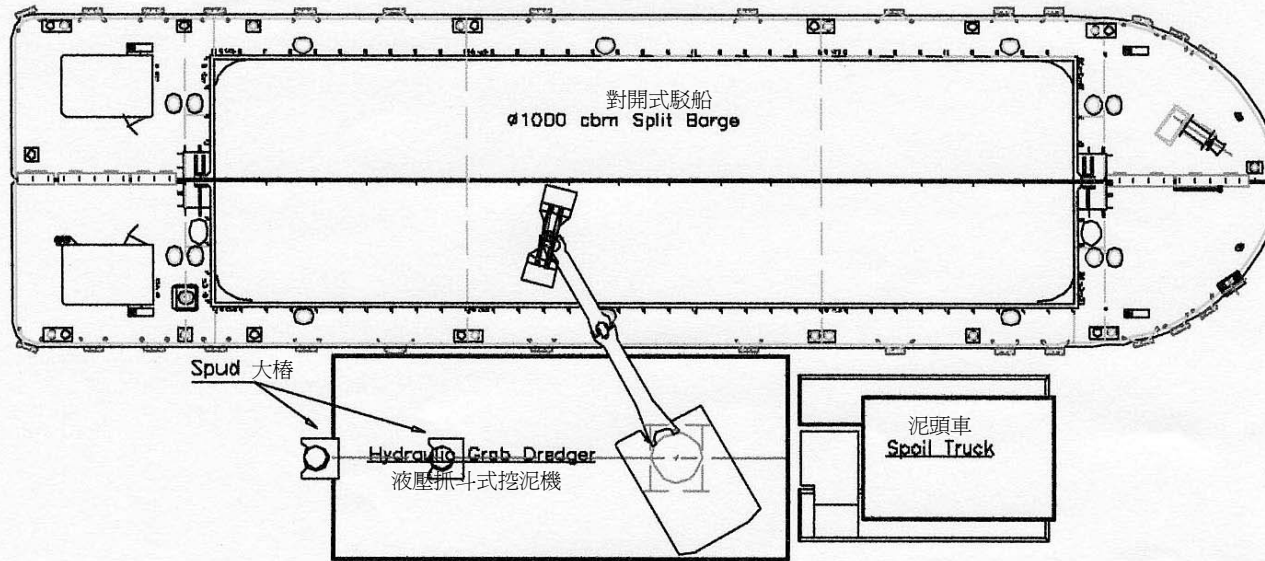
PLAN VIEW 俯視圖
