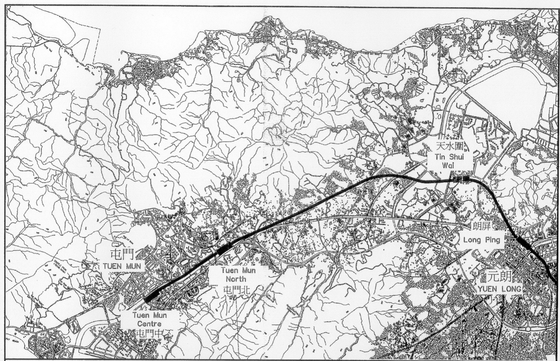
Figure 3 - Location and Alignment of the Project 圖3 - 工程項目的地點及線路
