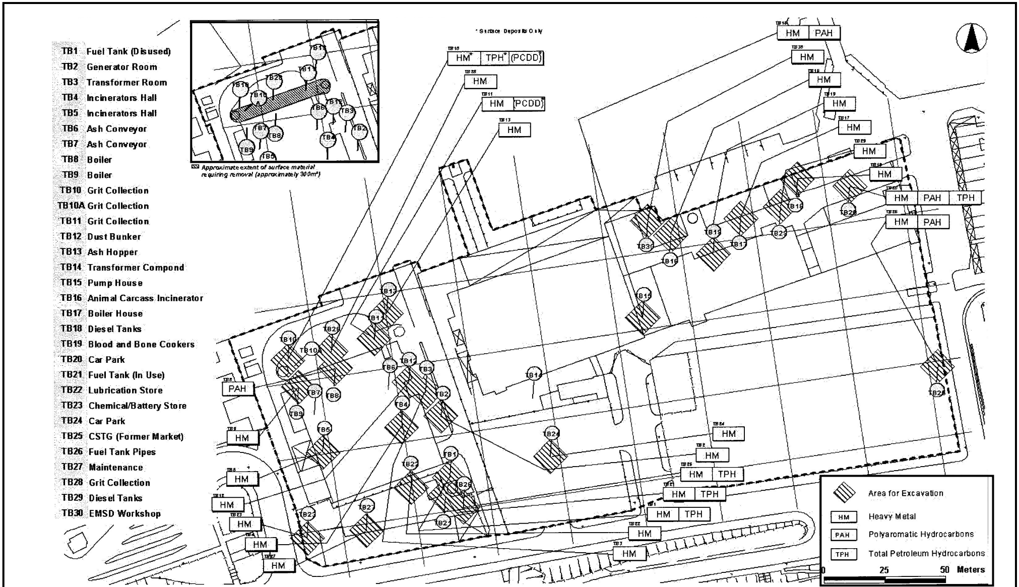
圖 7：鑽孔顯示受污染須作清理地點位置圖
