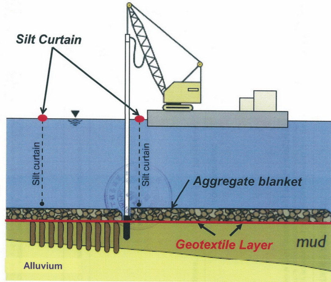
Schematic Section (N.T.S.)
