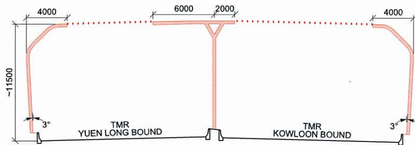
SECTION 14-14 SEMI-ENCLOSURE NM 21 (N.T.S.)
