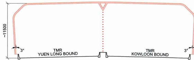
SECTION 15-15 FULL ENCLOSURE NM 24 (N.T.S.)
