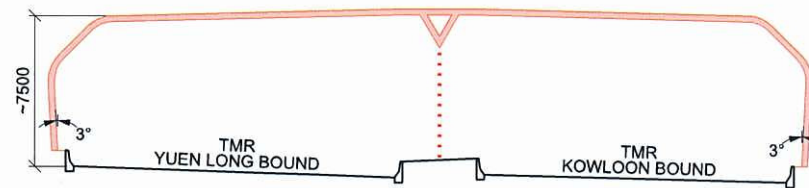
SECTION 5-5 FULL ENCLOSURE NM 8 (N.T.S.)
