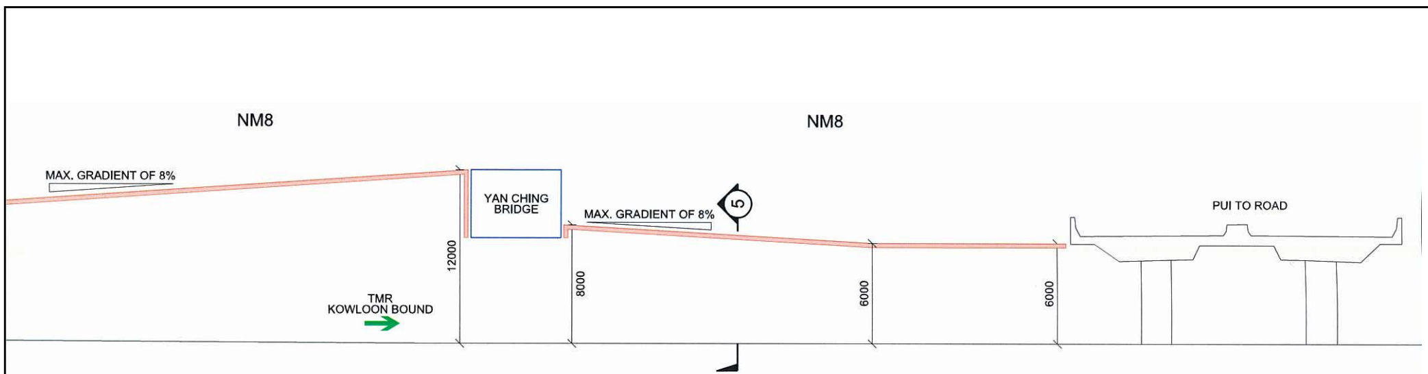
LONGITUDINAL SECTION ALONG TMR KOWLOON BOUND AT NM8 (N.T.S.)
