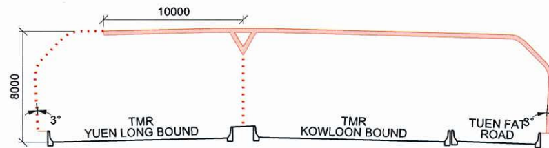
SECTION 9-9 SEMI-ENCLOSURE NM16 (N.T.S.)
