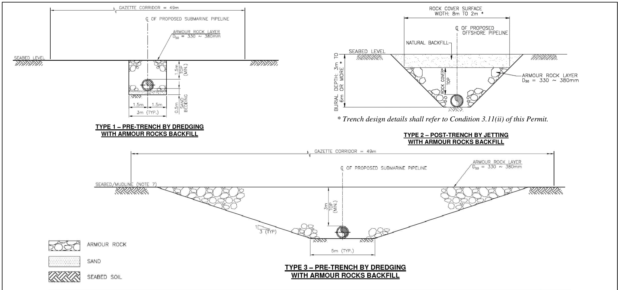
Figure 3 Black Point Gas Supply Project (Phase 1) 龍鼓灘燃氣供應項目（第一期） 圖三 Submarine Gas Pipeline – Trenching & Protection Details 海底輸氣管道的管道及保護設計
