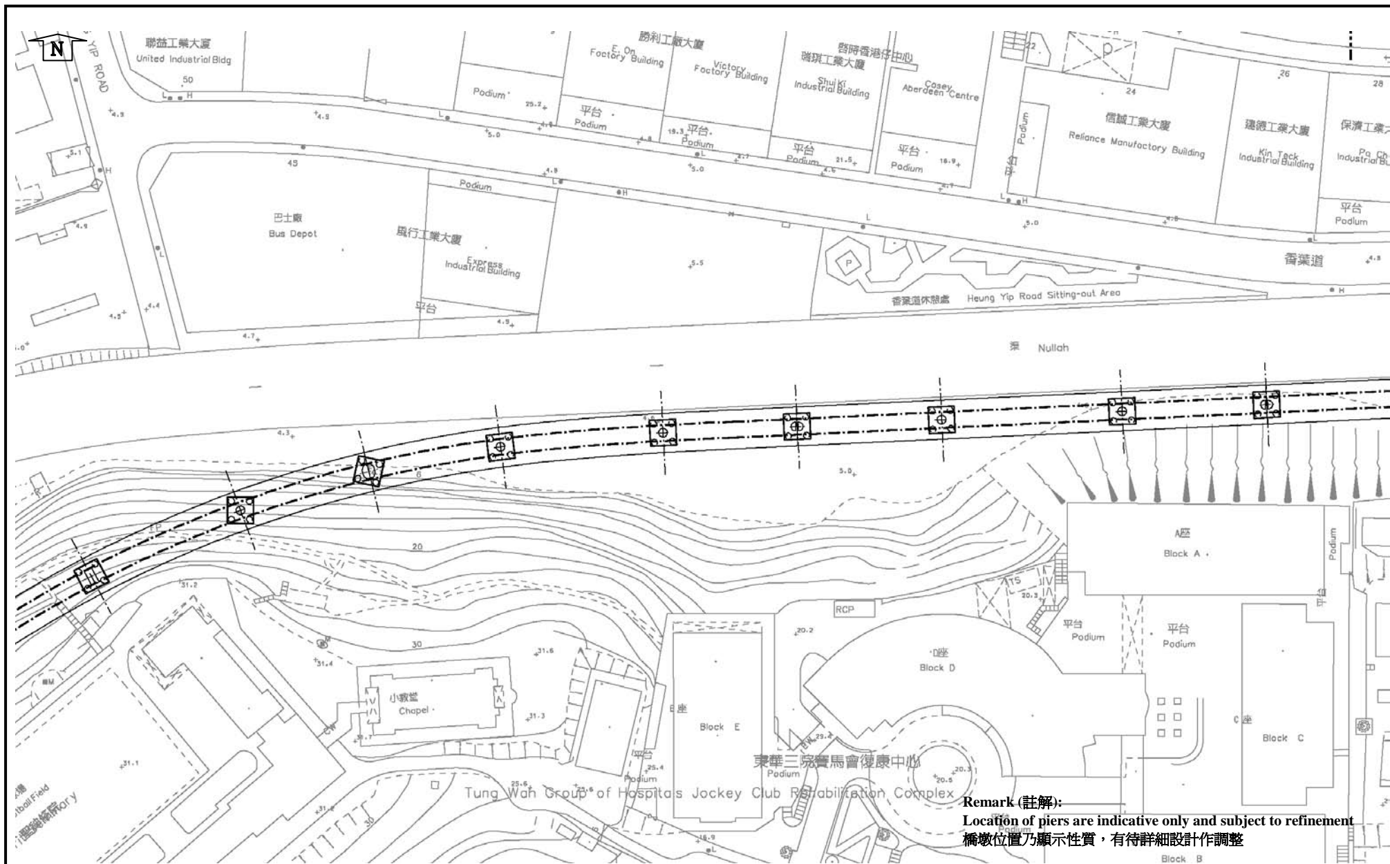
Figure 15d: Piers/Pier Foundations of Viaduct Section 圖 15d: 高架橋路段的鐵路橋橋墩/地基
