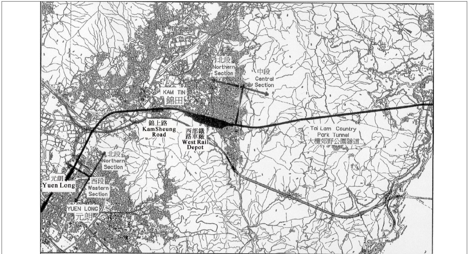
Figure 2 – Location and Alignment of the Project 圖二 – 工程項目的地點及線路
