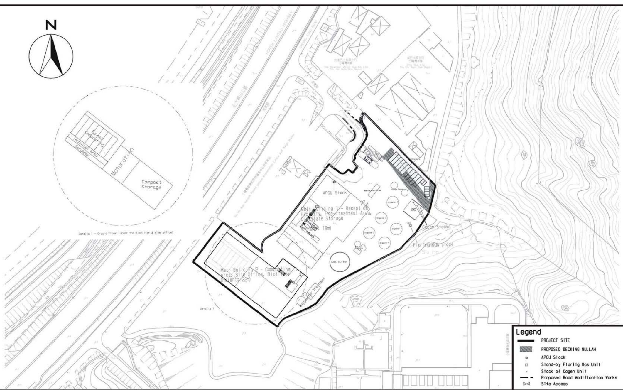
Figure 3 - Site Layout 圖 3 - 工地設計
