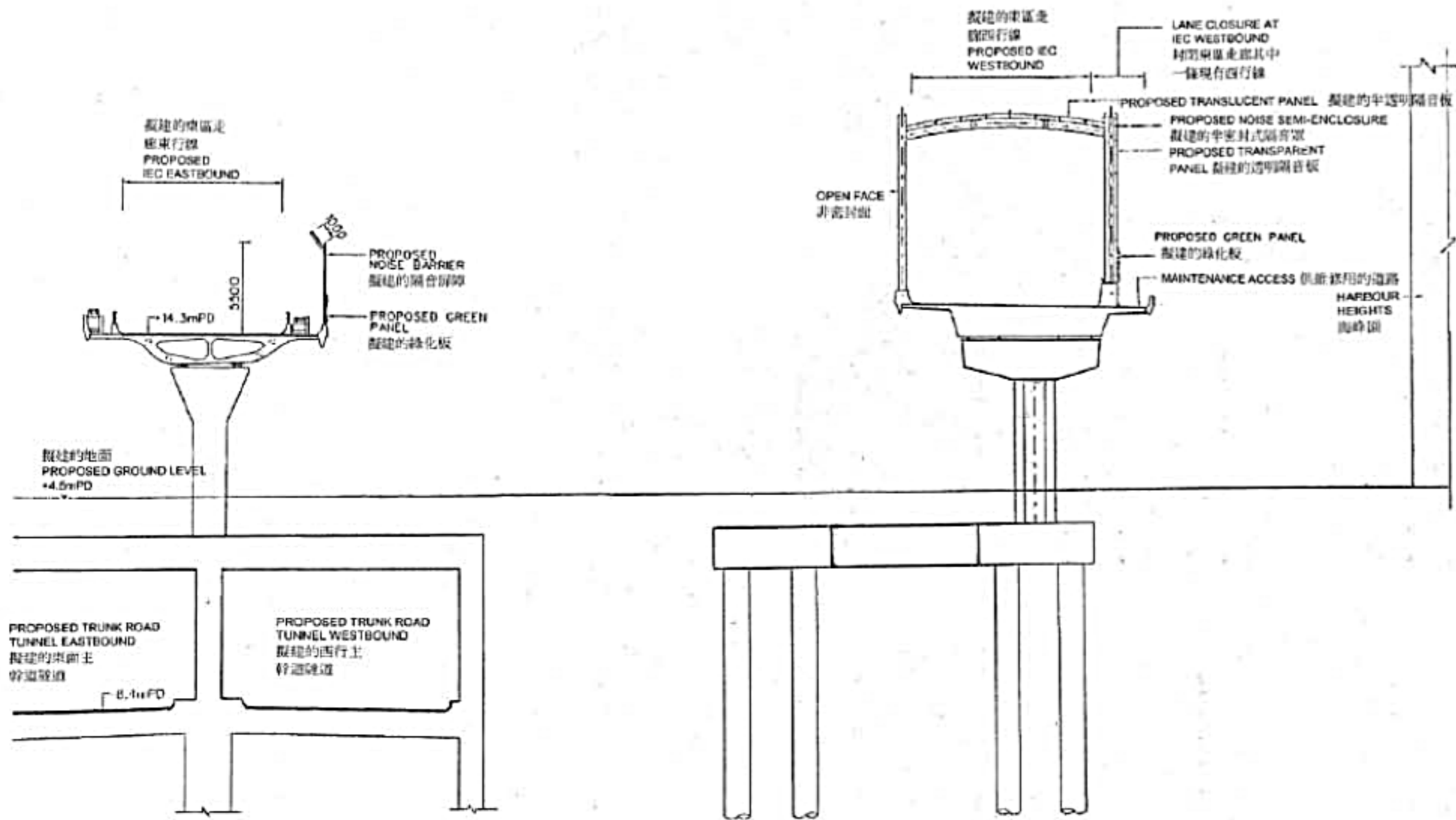
切面 A-A SECTION A-A
