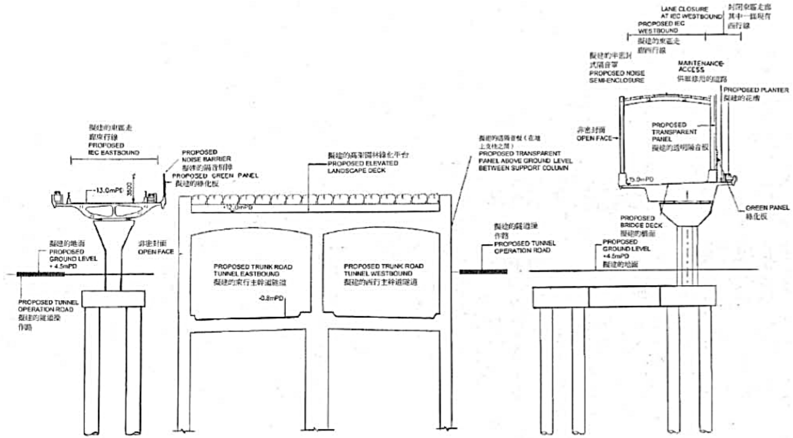
切面 B-B SECTION B-B
