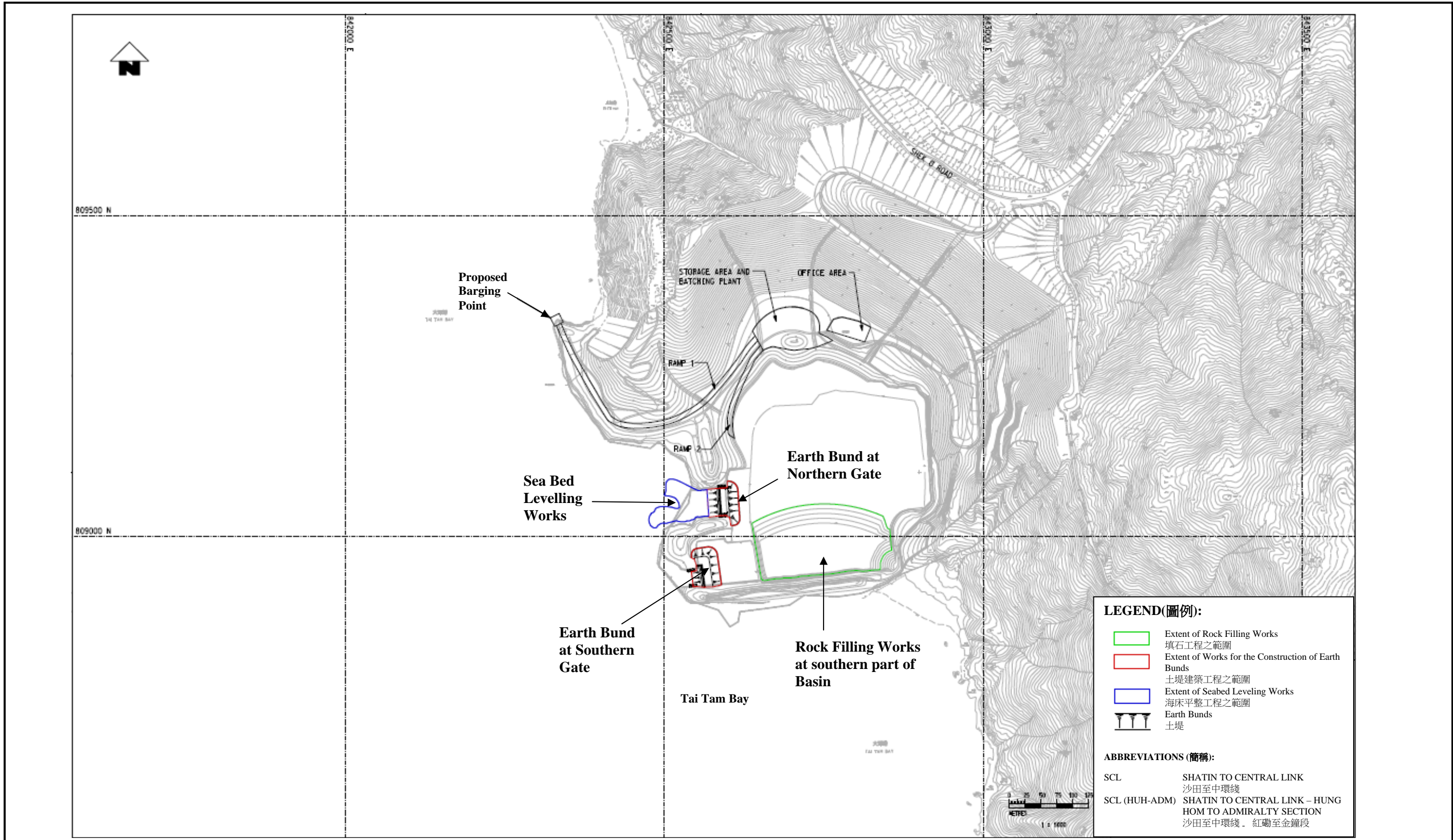
Figure 6: Works at Shek O Casting Basin 圖 石澳的沉管隧道預製件工場
