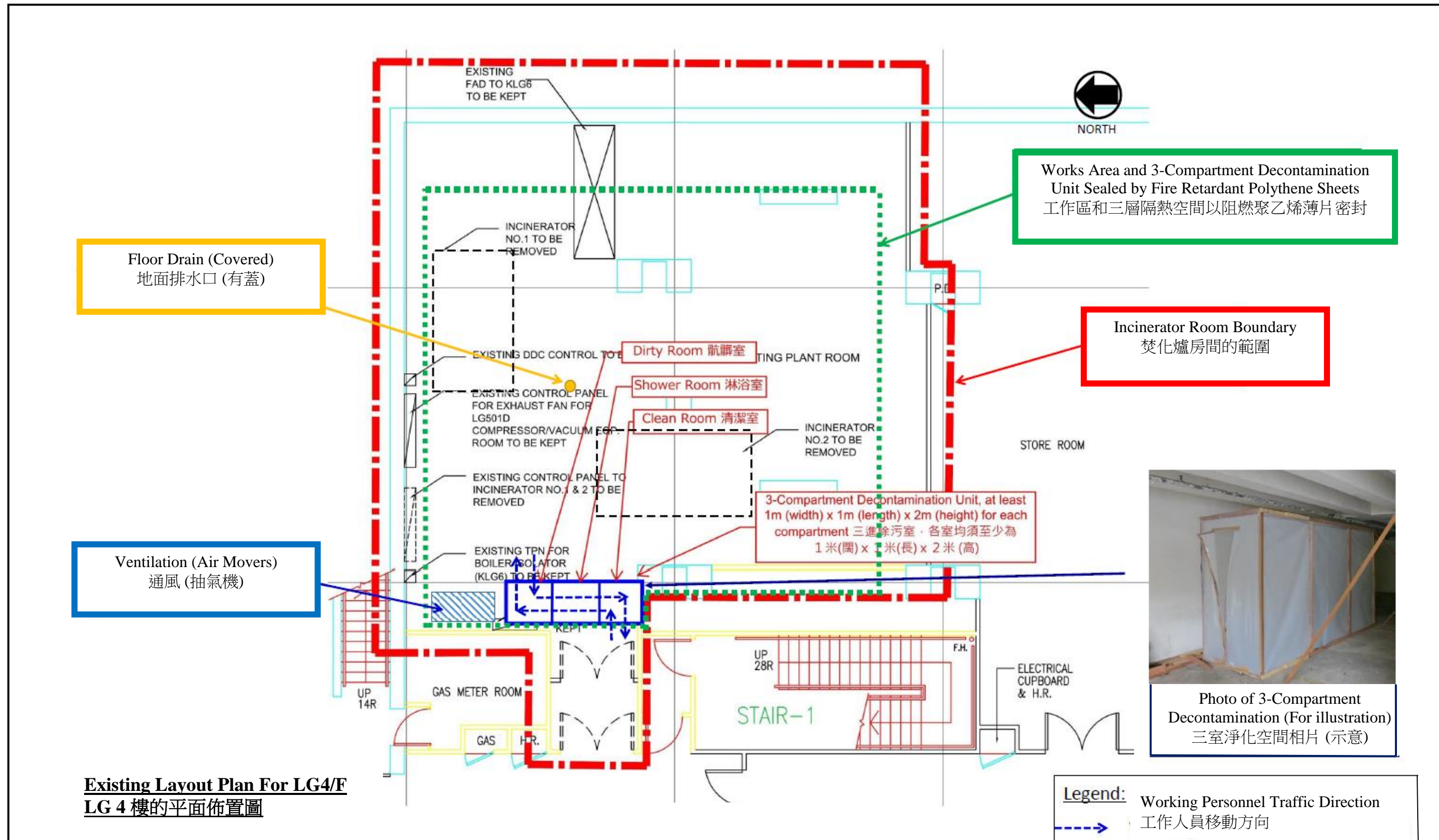
Figure 2: Floor Plan of the Incinerator Room in Block K 圖 2: 在 K 座焚化爐房平面圖
