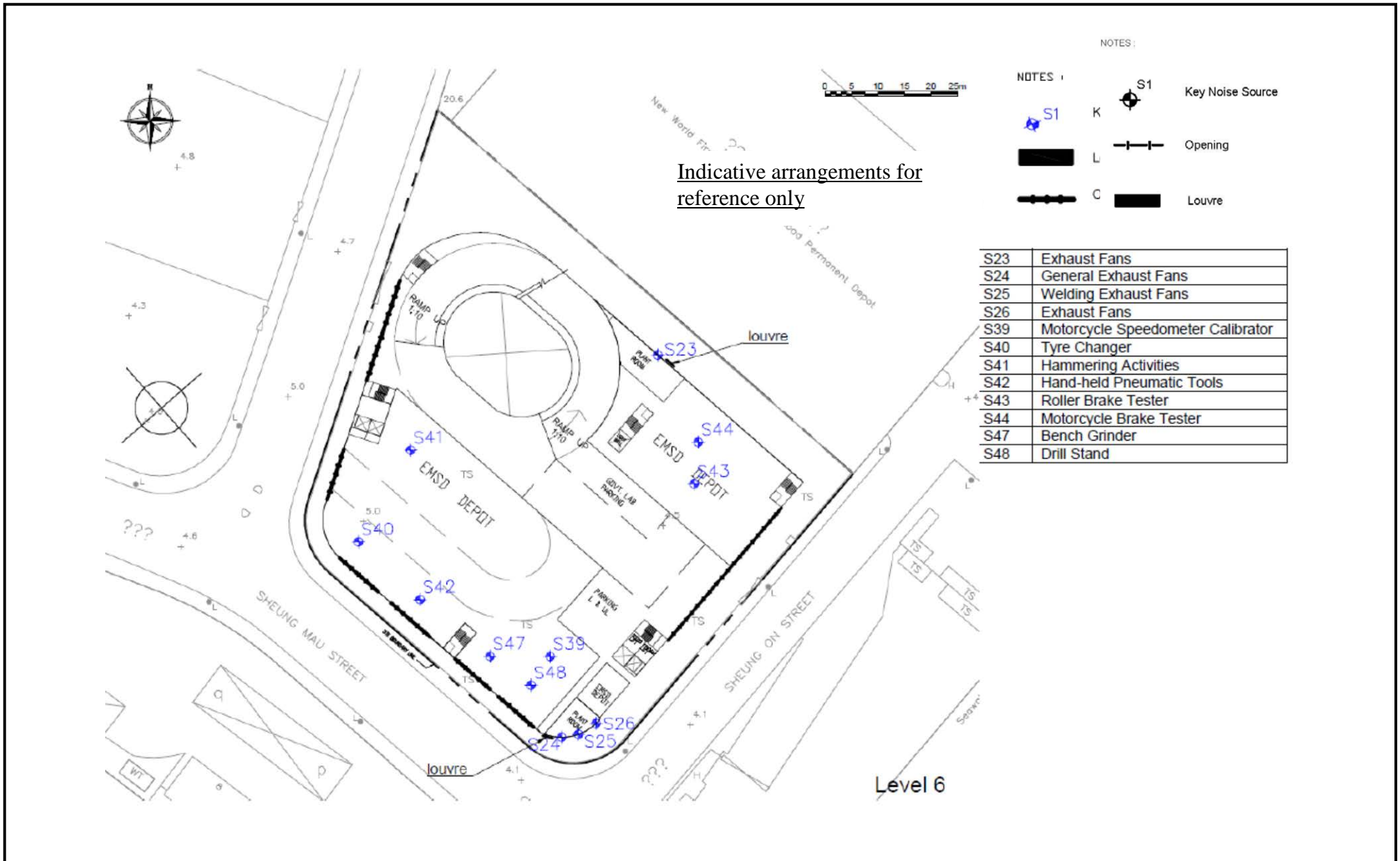
Figure 3: General Layout Plan of EMSD vehicle depot. 圖 3: 機電工程署修理車廠佈局圖
