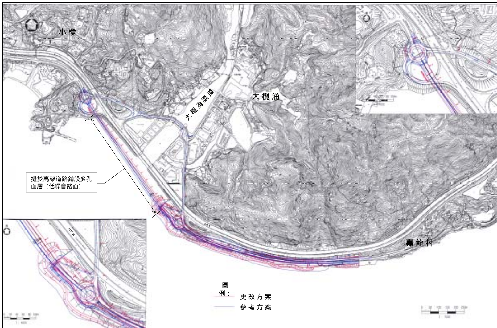
青山公路嘉龍村至小欖的改善工程 – 擬更改方案圖
